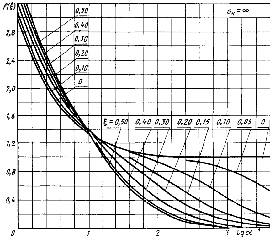
Рис. 17. Графики изменения функции жесткости f(\xi) проводника в зависимости от \lg(\alpha^{-1}) и координаты \xi точки приложения нагрузки для значений параметров \sigma_x = 0 и \sigma_{\kappa} = \infty
