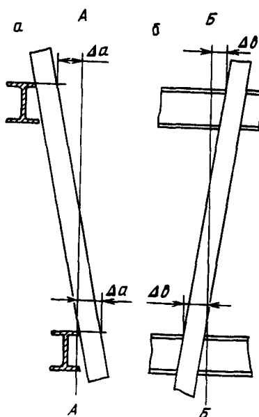
Рис. 19. Допускаемые отклонения проводников на двух смежных ярусах от вертикальной плоскости:
