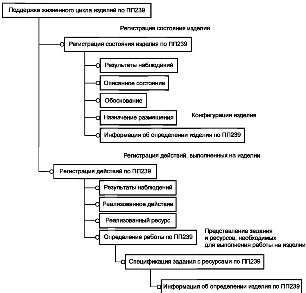
Рисунок 3 — Основная часть иерархии модулей
