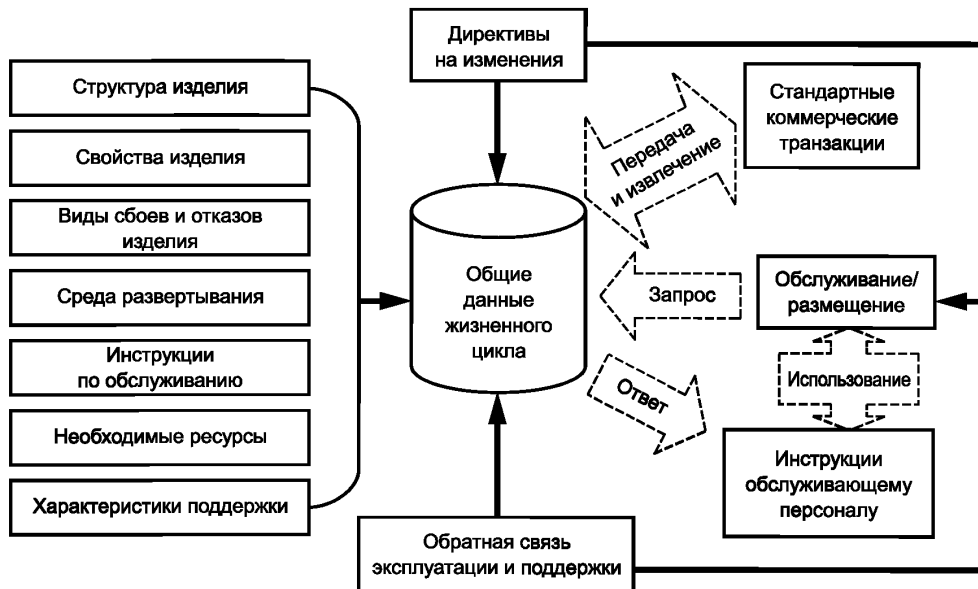
Рисунок 1 — Визуальное представление ПЖЦИ
