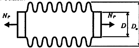
Рисунок 8.2. - Схема приложения распорных усилий в осевом компенсаторе
