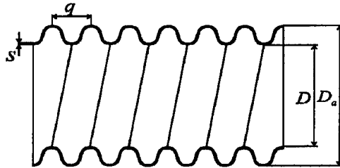
Рисунок 11.1. - Элемент гофрированной трубы
