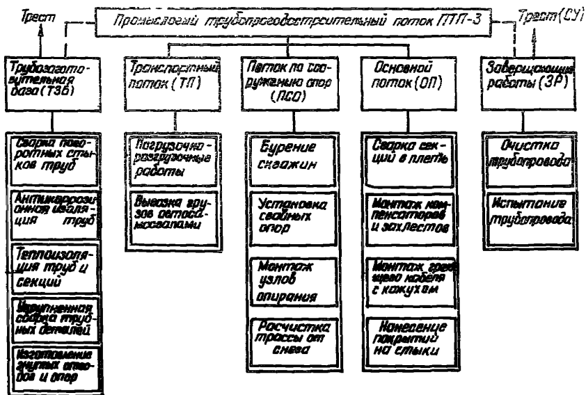
Рис.3. Организационная структура промышленного трубопроводостроительного потока по строительству водоводов и канализационных сетей
