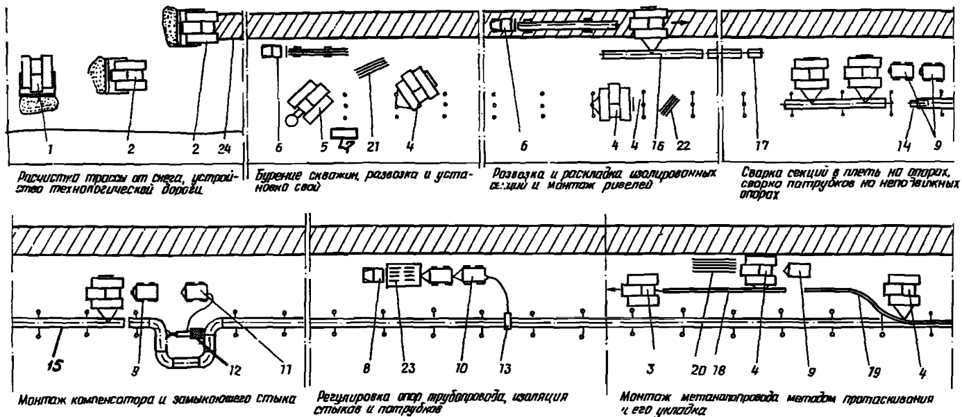
Рис.4. Поточно-индустриальный метод строительства газопроводов-шлейфов на Ямбургском ГКМ:
