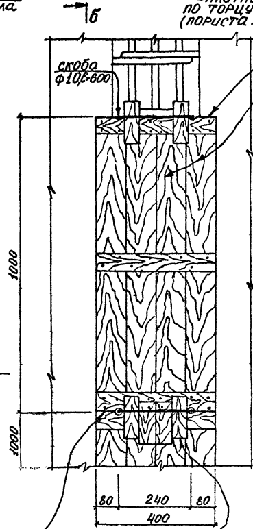
Узел крепления опалубки к арматуре стыка
