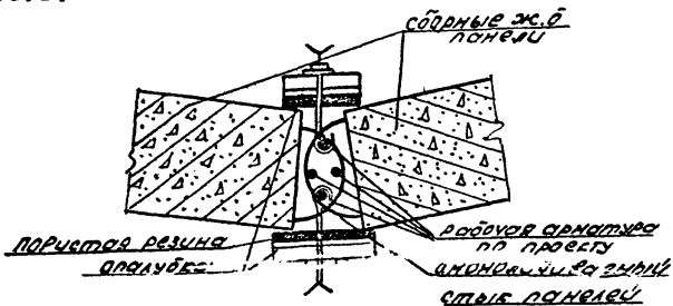
Рис. 2. Деталь монолитного стыка
