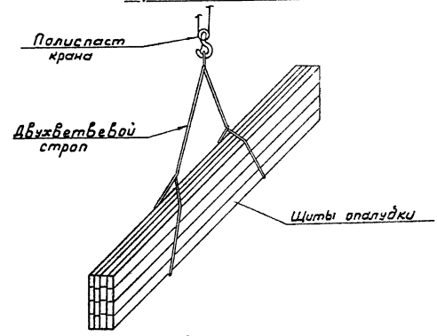
Двухветвевой строп
