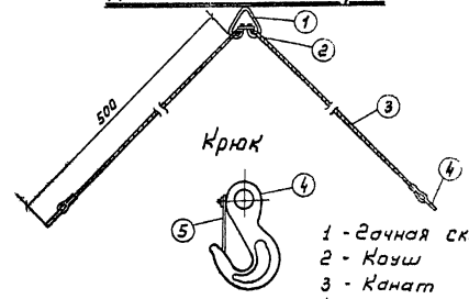
Двухветвевой строп
