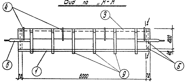
План
