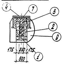
Разрез 1-1
