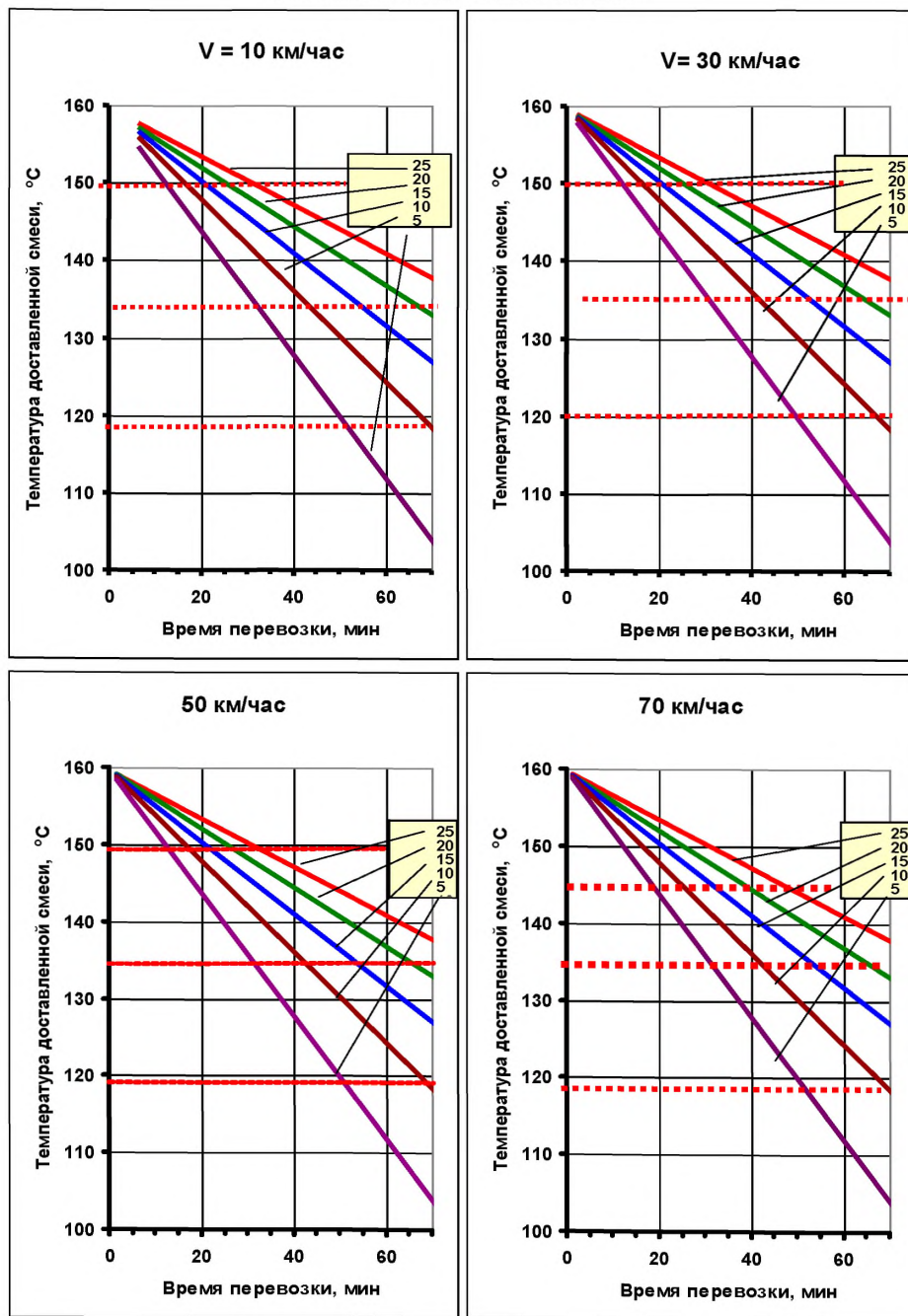
Рисунок В.1 Время перевозки горячей асфальтобетонной смеси в автомобилях самосвалах (при температуре отгрузки t_{\text{нач}} = 160 °С)
