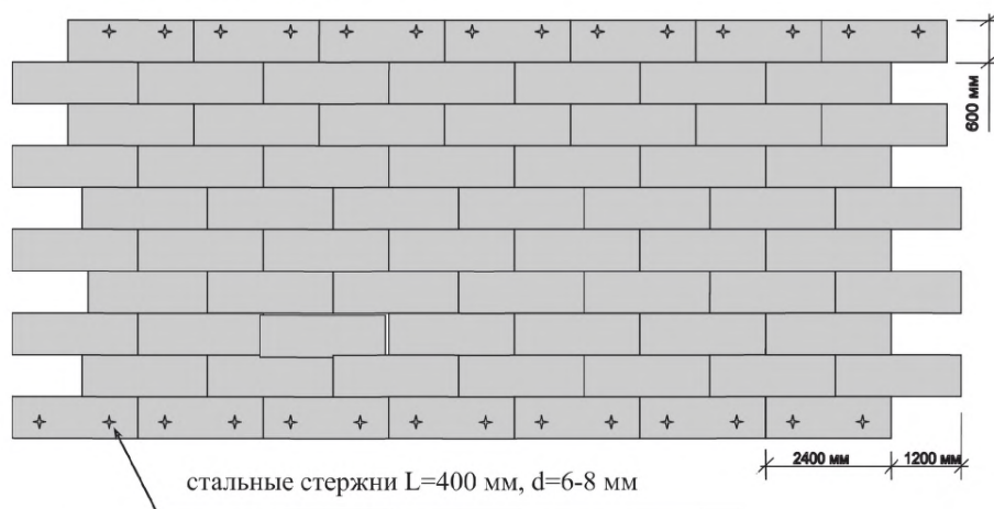
Рисунок 5 – Раскладка вспененных геоплит в теплоизоляционном слое
