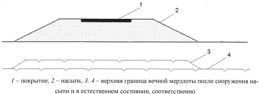
Рисунок 3 – Схема дорожной конструкции, запроектированной по второму принципу
