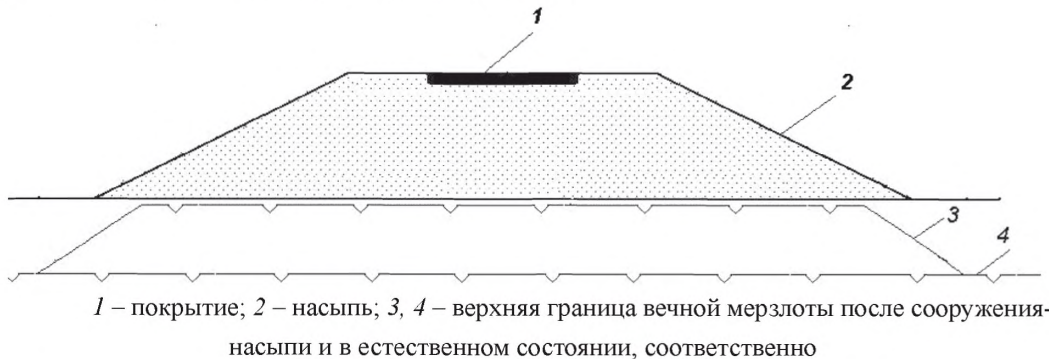
Рисунок 2 – Схема дорожной конструкции, запроектированной по первому принципу
