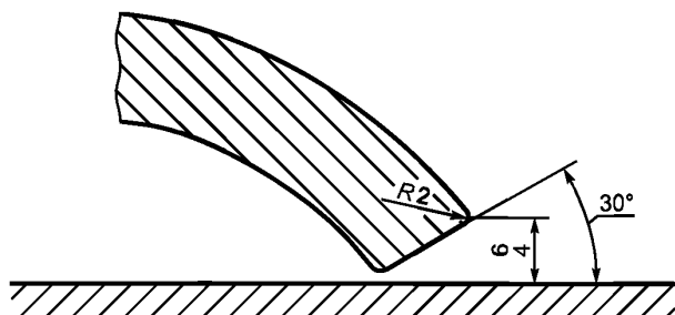
Рисунок 11 — Вариант 2: конструкция кромки ограждения со стороны загрузки
