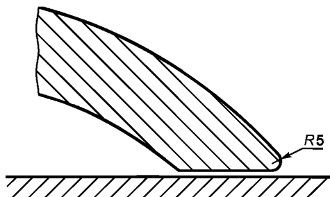
Рисунок 10 — Вариант 1: конструкция кромки ограждения со стороны загрузки
