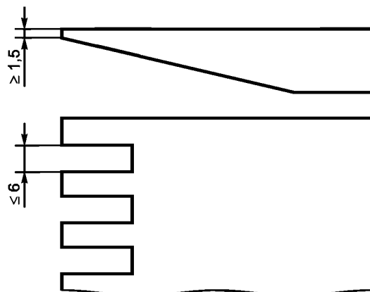
Рисунок 6 — Пример кромки стола с пазами
