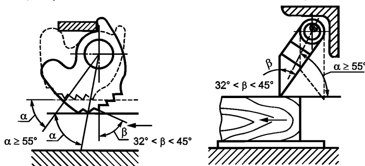
Рисунок 4 — качающиеся элементы (зубчатые секторы)
