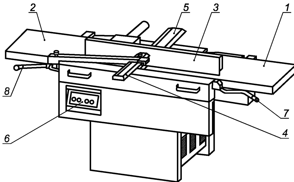
Рисунок 1а) — Пример использования фуговально-рейсмусового станка при фуговании
