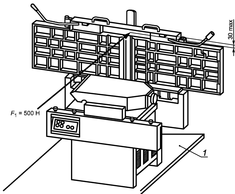
Рисунок D.2 — Испытание на устойчивость передвижных станков (установка при рейсмусовании)
