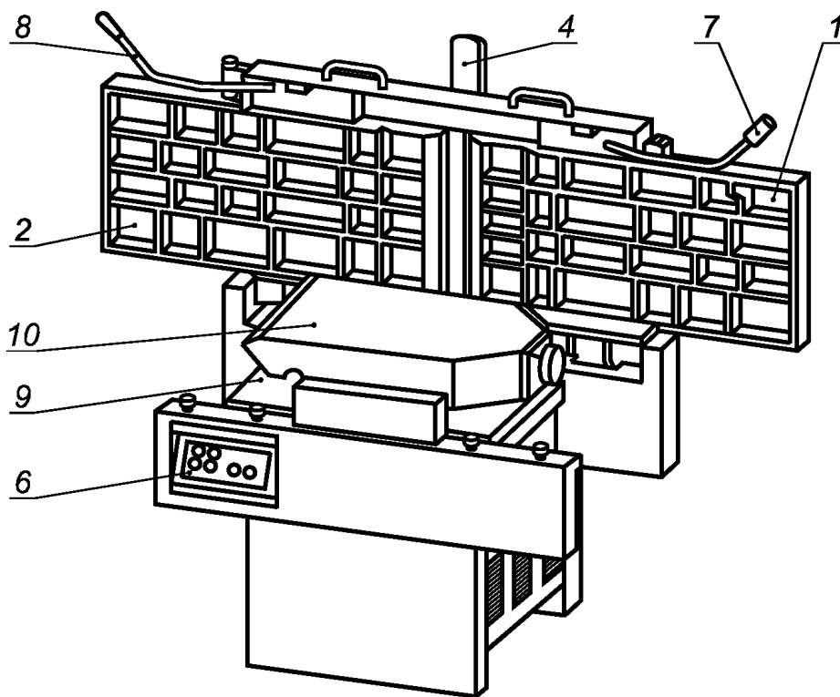
Рисунок 1б) — Пример использования фуговально-рейсмусового станка при рейсмусовании
