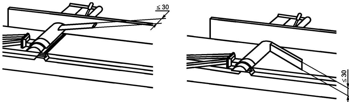
Рисунок 9 — Примеры нагружающих устройств
