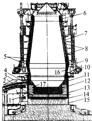
Рисунок Ж.1 – Углеродистая кладка лещадки и горна
