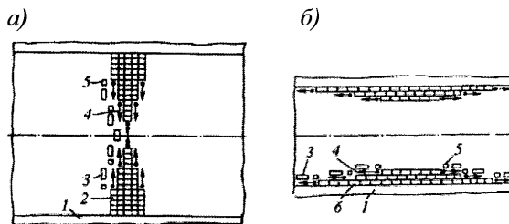
1 – пятовая балка; 2 – кольцо; 3 – штабеля изделий; 4 – огнеупорщики; 5 – ящики с раствором; 6 – первый ряд свода
