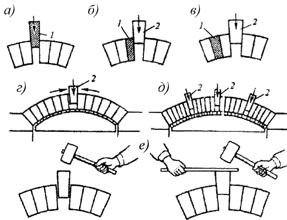
a, б – неправильно; в – правильно; г – малый пролет; д – пролет шириной более 3 м; е – забивка замка; 1 – тесанные изделия; 2 – замок
