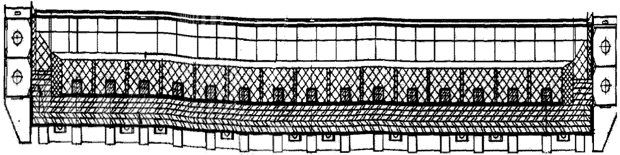
Рисунок Ж.10 – Схема катодной футеровки (продольный разрез)
