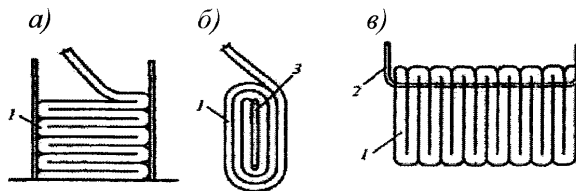
а – укладка гофрированием; б – укладка на рамку; в – готовый элемент; 1 – рулонный материал; 2 – элемент крепления; 3 – рамка
