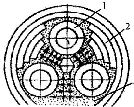
1 – шаблон; 2 – огнеупорная кладка; 3 – набивка (стрелки – направление хода трамбовок при чередовании слоев набивки)
