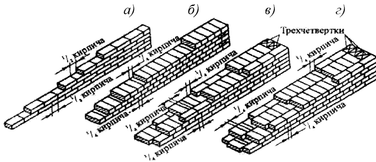
Рисунок 3 – Кладка прямых стен
