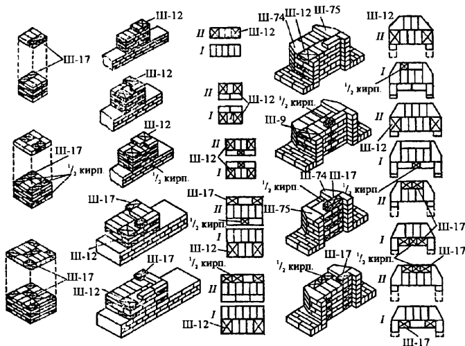
Рисунок 7 – Перевязка швов при кладке прямоугольных простенков
