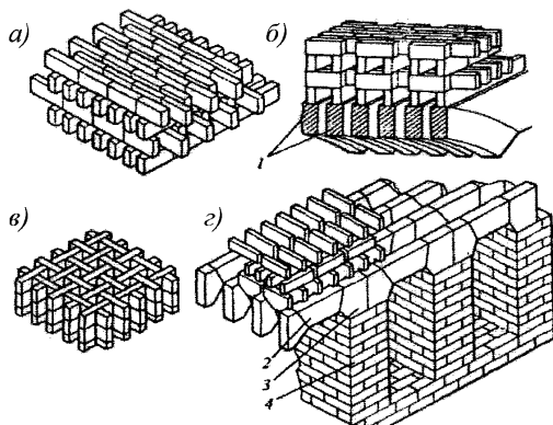
a, б – с открытыми каналами; в – с закрытыми каналами; з – фрагмент поднасадочного устройства; 1 – поднасадочная арка; 2 – распорное изделие; 3 – пята; 4 – поднасадочная стена
