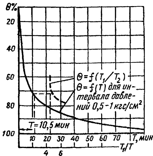
Рис. 15. Кривая консолидации
