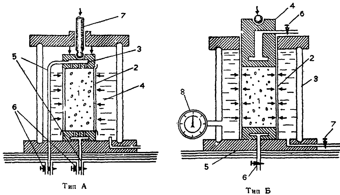
Рис. 19. Схемы стабиметров
