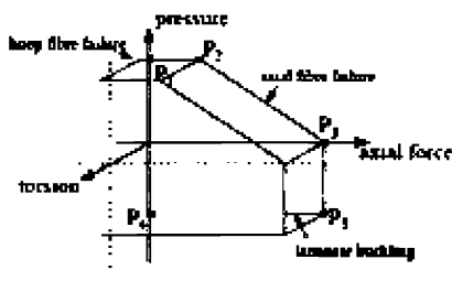
Рис. 4 Общая поверхность разрушения трубы райзера из ПКМ, нагруженного внешним давлением, осевой силой и крутящим моментом.
