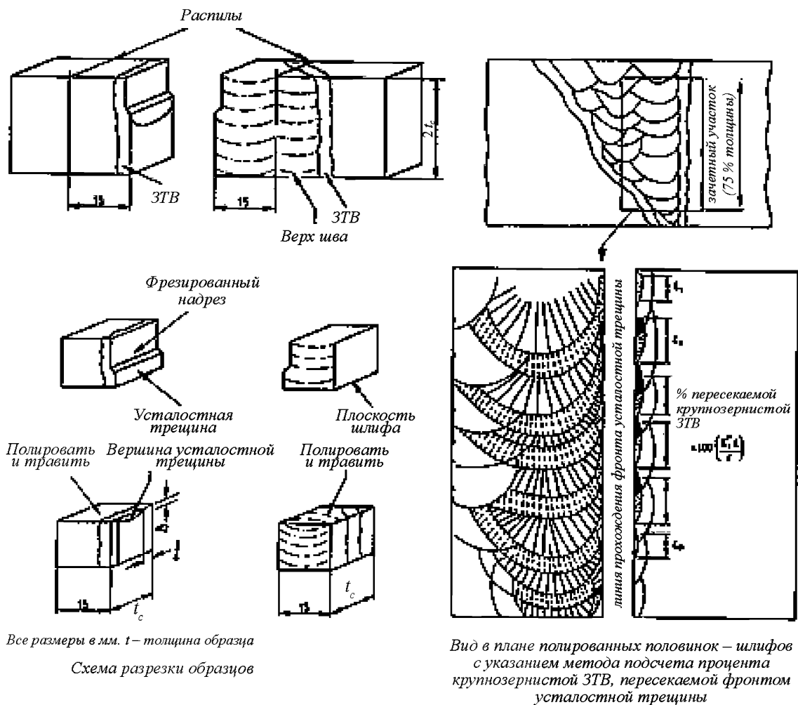
Рис. 5.4.4.8 Порядок металлогрфического исследования после испытания
