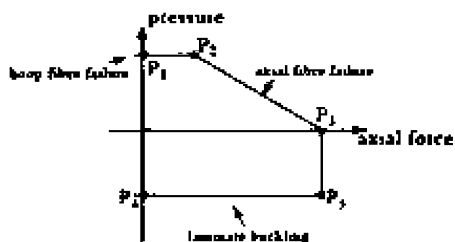
Рис. 3 Поверхность разрушения трубы райзера из ПКМ, нагруженного внутренним давлением и осевой силой.
