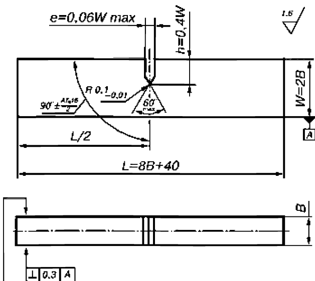
Рис. 2.2 Предпочтительный тип образцов для испытаний на СТOD
