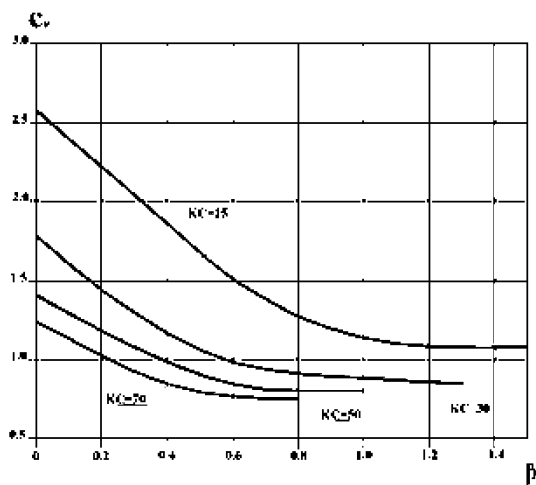
Рис. 9-3 Коэффициент c_c в зависимости от коэффициента \beta
