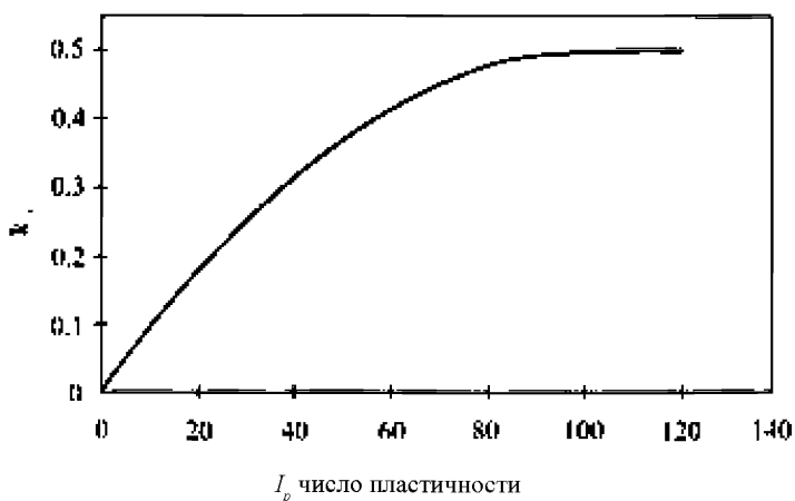
Рис. 3.2.3 Зависимость показателя степени k_p от числа пластичности I_p
