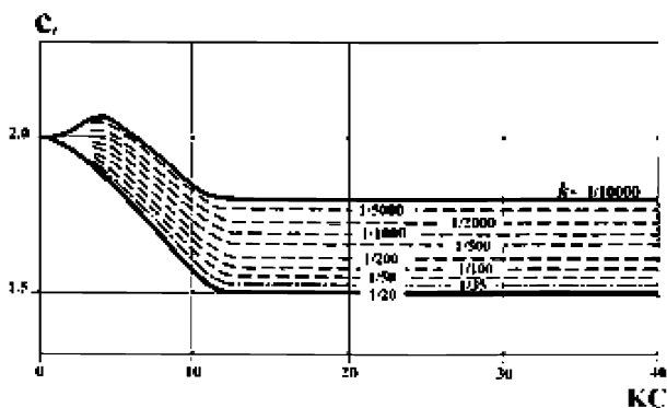
Рис. 1-2 Коэффициент c в зависимости от числа Кюлегана-Карпентера KC и относительной шероховатости k поверхности трубопровода
