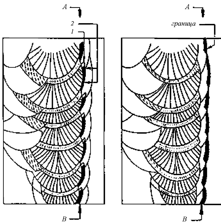
а) повторно нагретые межкритически (1) и субкритически (2) районы ЗТВ с крупным зерном
