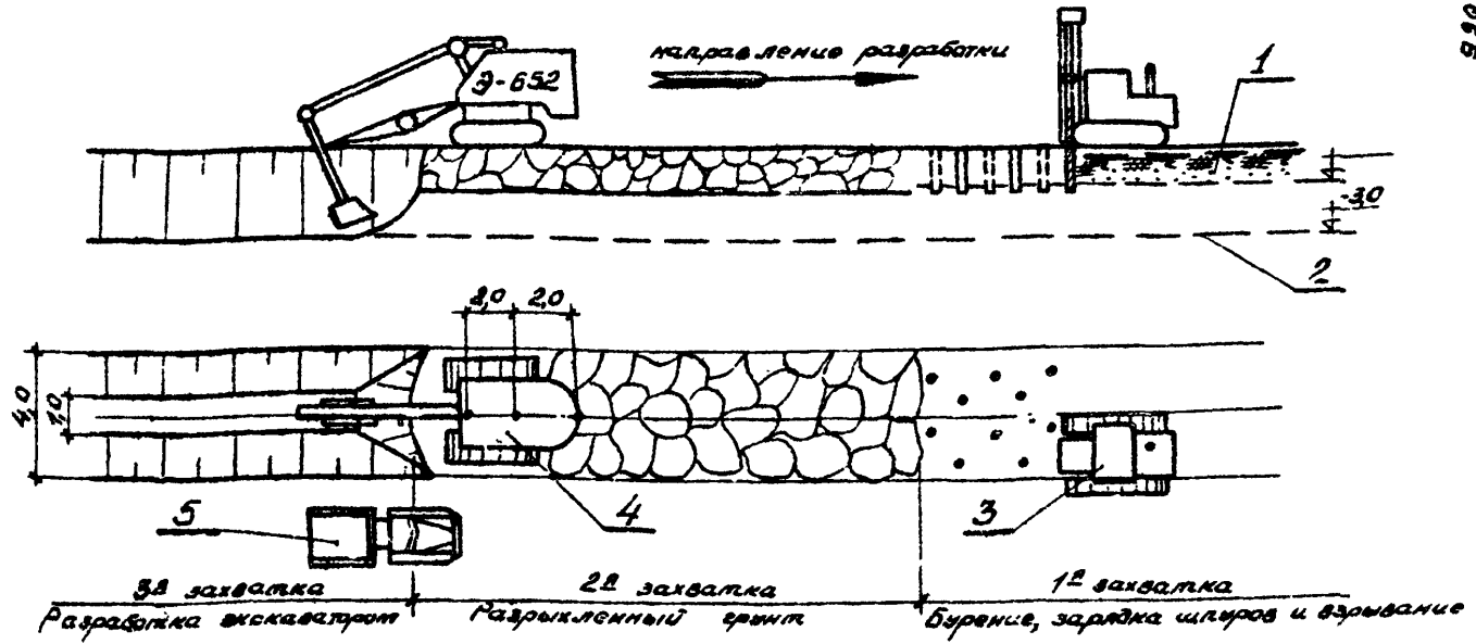
рис. 3 Схема разработки траншеи при рыхлении мерзлого грунта бурно-взрывным способом
