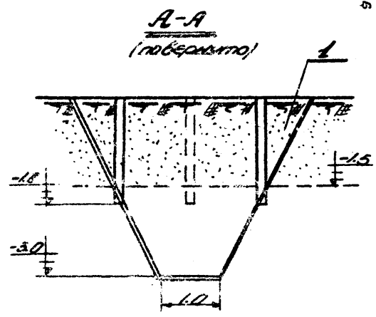
рис 5 Система расположения шпуров при проходе траншеи
