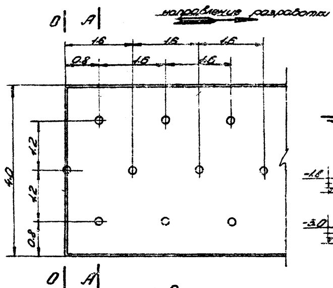
рис 5 Система расположения шпуров при проходе траншеи
