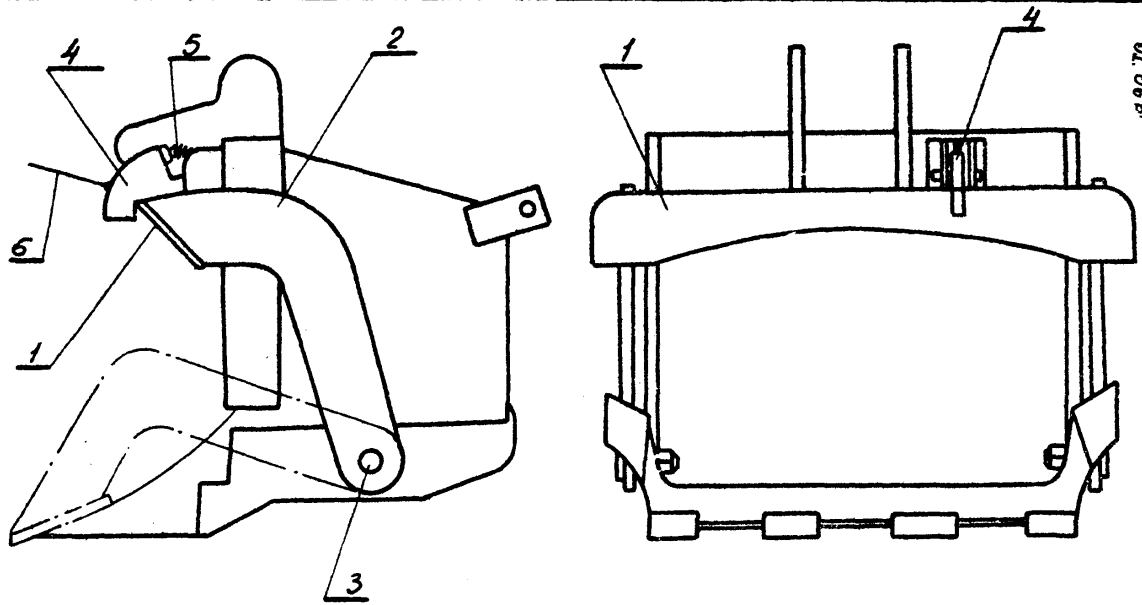
Рис. 2 Струз для зачистки дна траншеи экскаватором 1- Нож струза; 2- упорные штанги; 3- цапфа; 4- замок-защелка 5- пружина; 6- тросик
