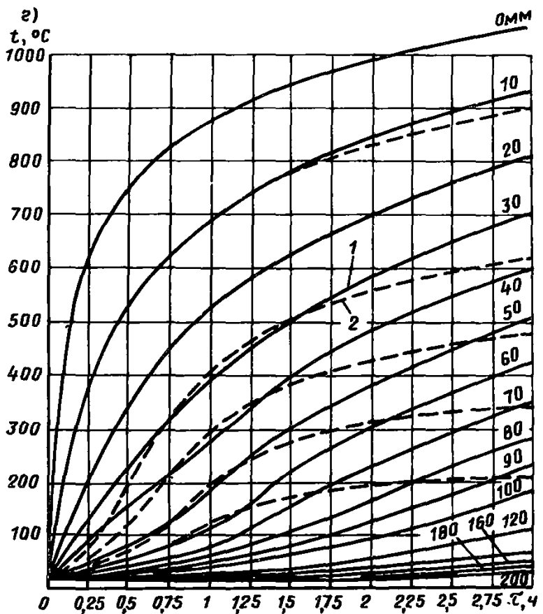
Рис. 1. График зависимости температуры t °С от времени \tau в отдельных точках плиты
