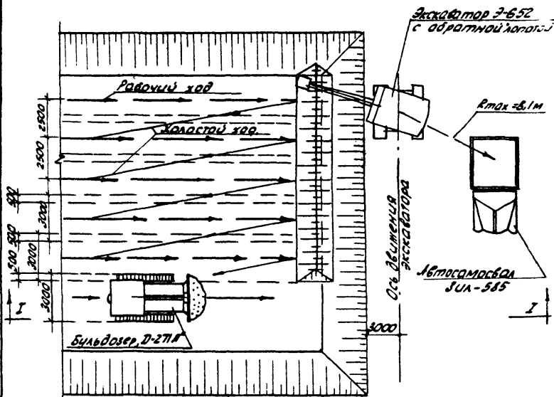
Схема зачистки дни котлована бульдозером «Д-271А»
