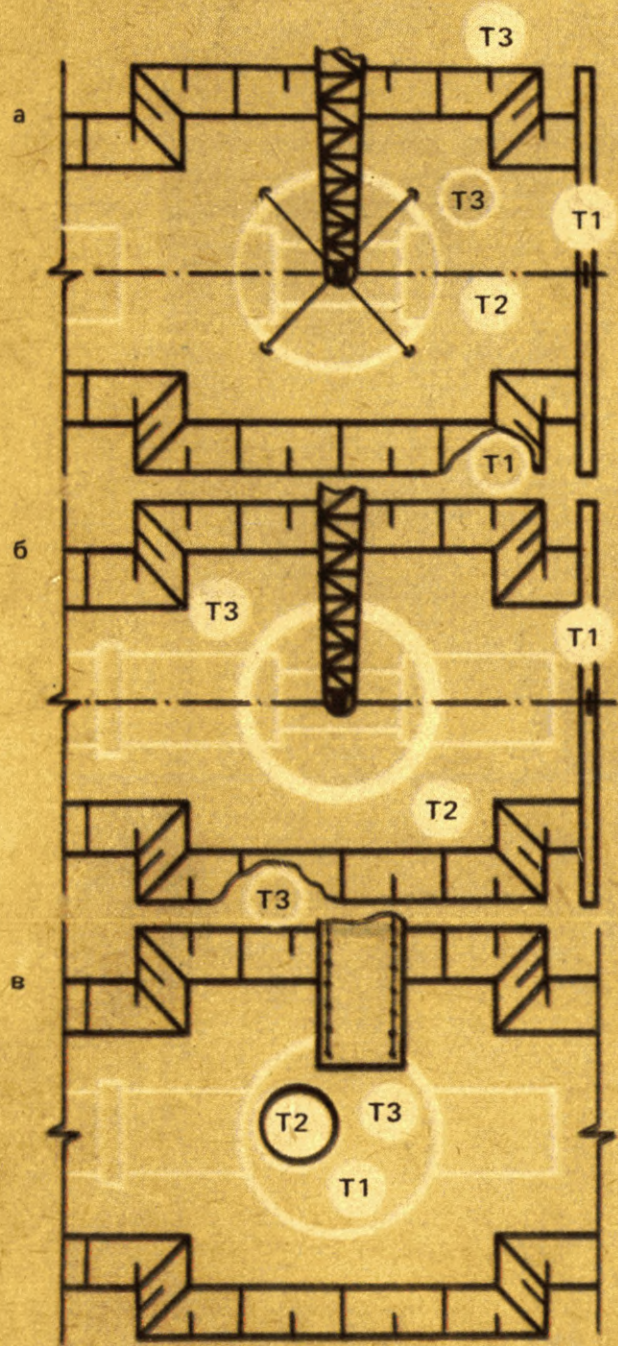
Схема организации рабочего места а — подготовительные работы и установка лоткового блока; б — установка отдельных колец; в — установка лестницы и люка Т1, Т2, Т3 - рабочие места трубоукладчиков
