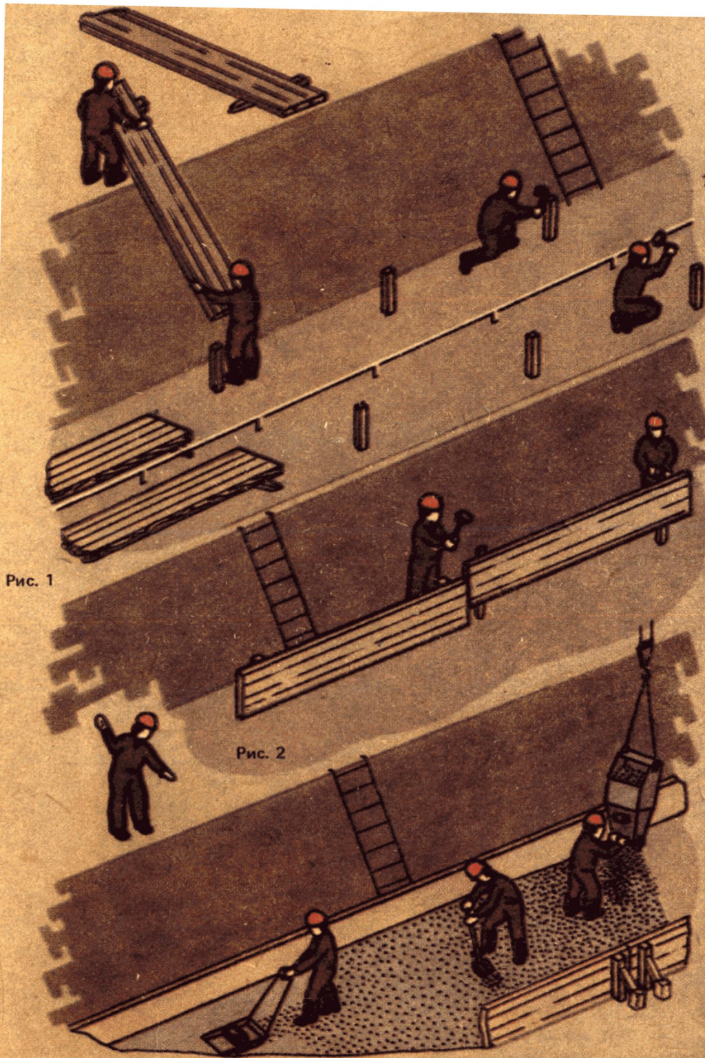
Схема организации рабочего места а — установка опалубочных щитов; б — устройство бетонной подготовки; в — армирование основания 1 — щиты опалубки; 2 — бадья с бетонной смесью; 3 — кран; 4 — арматурные каркасы Т1, Т2, Т3, Т4 — рабочие места трубоукладчиков
