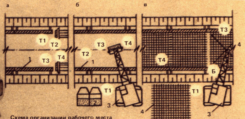
Схема организации рабочего места а — установка опалубочных щитов; б — устройство бетонной подготовки; в — армирование основания 1 — щиты опалубки; 2 — бадья с бетонной смесью; 3 — кран; 4 — арматурные каркасы Т1, Т2, Т3, Т4 — рабочие места трубоукладчиков
