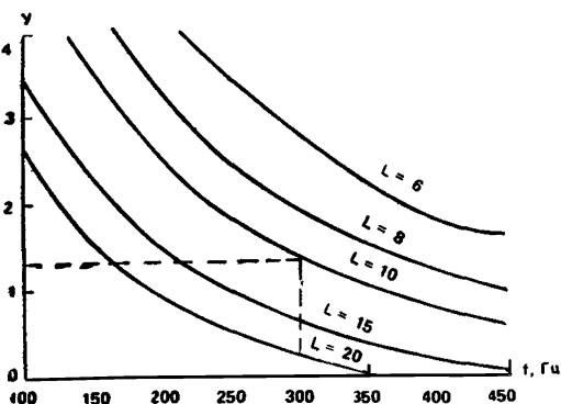
Рис. 3. Частотная зависимость мнимой компоненты Y=Y_{\Pi}-Y_2 импеданса однослойного резонатора с тканью ЭЗ-100, рассчитанная при различных значениях глубины воздушной полости
