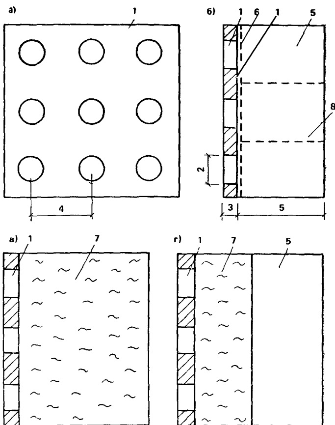
Рис. 1. Однослойный резонатор
