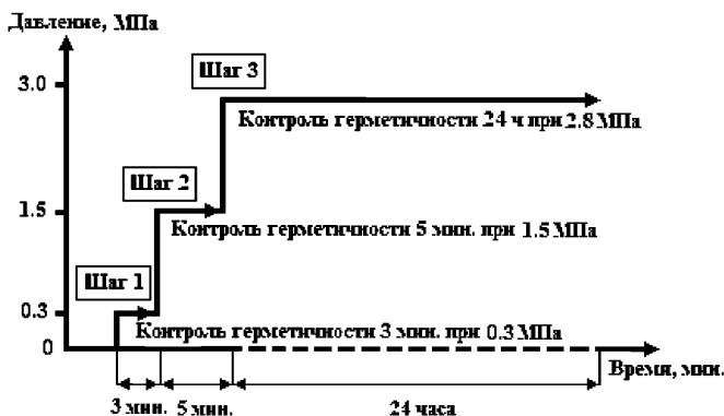
Рисунок 1 - Проверка герметичности азотом хладагентов R 22, R 407C
