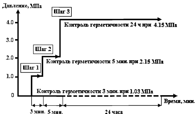
Рисунок 2 - Проверка герметичности азотом хладагента R 410A
