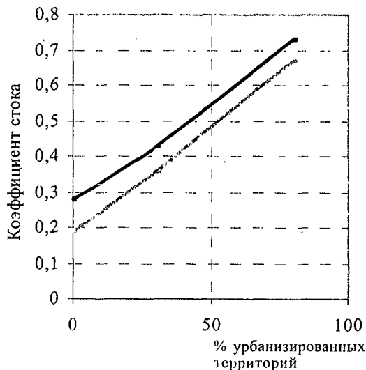
Рис. 2. Зависимость коэффициентов годового полного и поверхностного стока от площади урбанизированных территорий (в процентах от общей площади): ———— – коэффициент полного стока; - - - - - – коэффициент поверхностного стока
