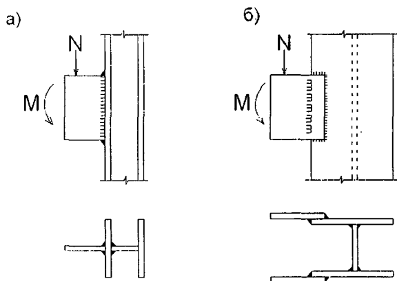
а — перпендикулярной; б — параллельной плоскости расположения швов
