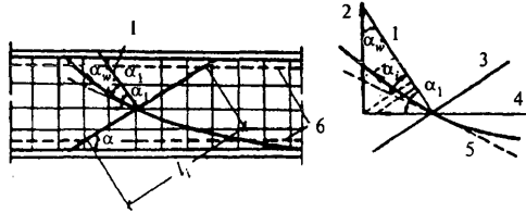
1 — нормали; 2 — хомут; 3 — наклонное сечение; 4 — продольная арматура; 5 — касательная к пучку; 6 — вут Рисунок 7.9 — Проекции усилий в поперечной арматуре на нормаль к наклонному сечению
