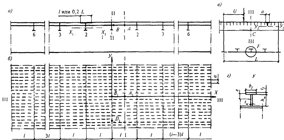
1, 2, 3, ... i – номер поперечного ребра верхней плиты a – продольный разрез; b – план; c – поперечный разрез; d – ребро нижней плиты
