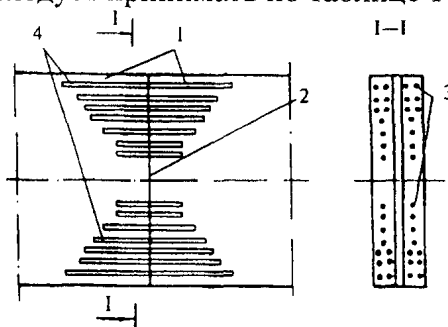
Рисунок 10.1 — Клеештыревой стык
