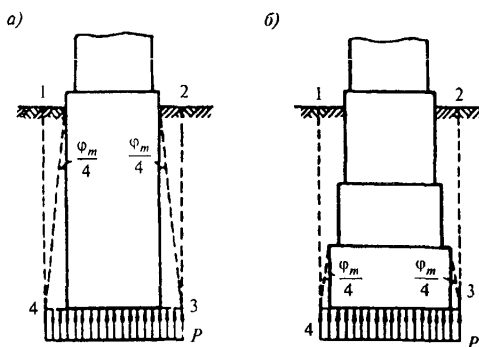
а – без уступов; б – с уступами
