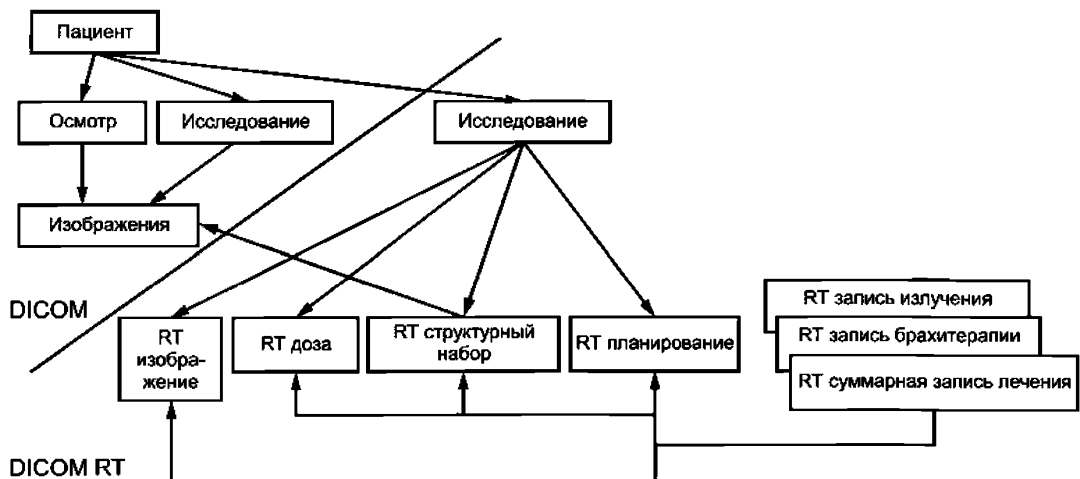
Рисунок 2 — Информационная модель DICOM (с расширением на RT)
