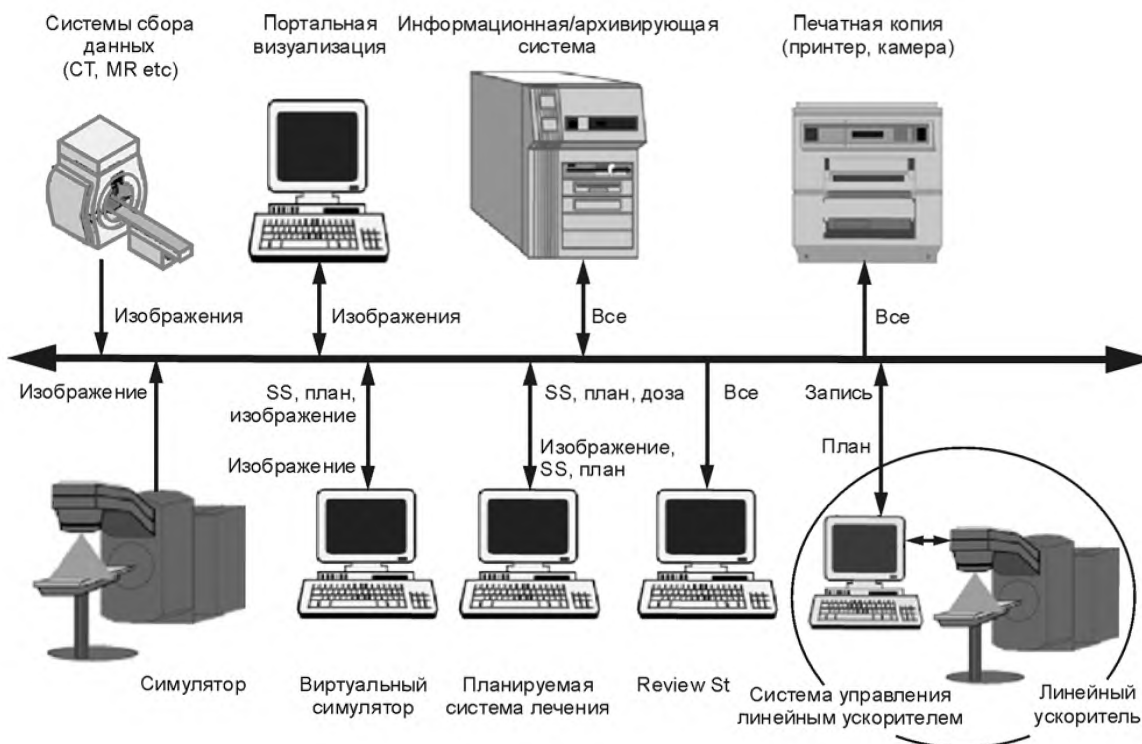
Рисунок 3 — Пример DICOM (включая объекты RT)
