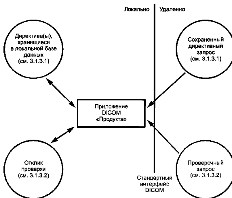
Рисунок 4 — Модель применения «Продукта»
