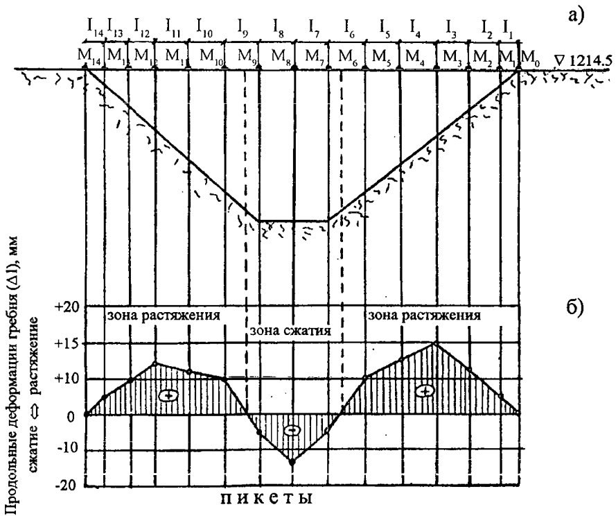
Рис.3.14. Эпюра продольных деформаций гребня плотины:
