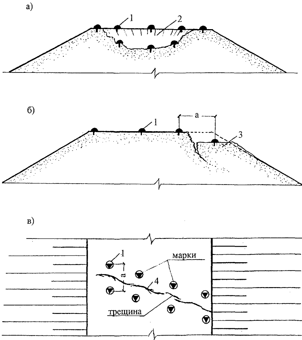
Рис.3.5. Схема размещения временных высотных марок для контроля: a – просадки; б – оползня; в – трещины; 1 – поверхностная марка; 2 – воронка проседания; 3 – массив оползня; 4 – трещина
