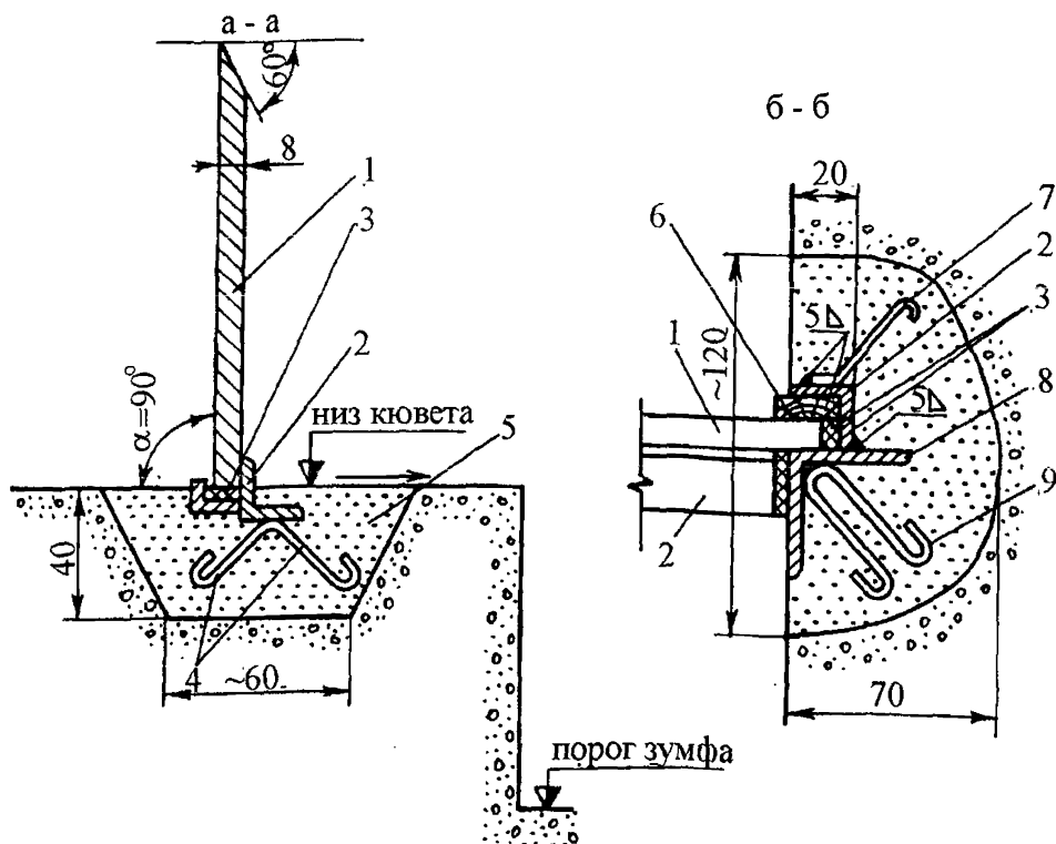
Пл. 13. Установка мерного треугольного водослива на водоотводящих кюветах:
