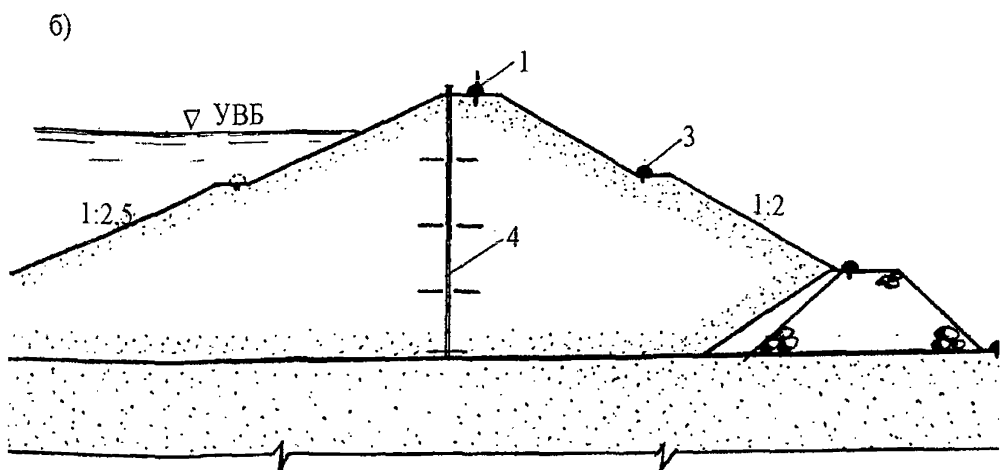
Рис.3.3. Принципиальные схемы размещения геодезических марок на грунтовых плотинах:
