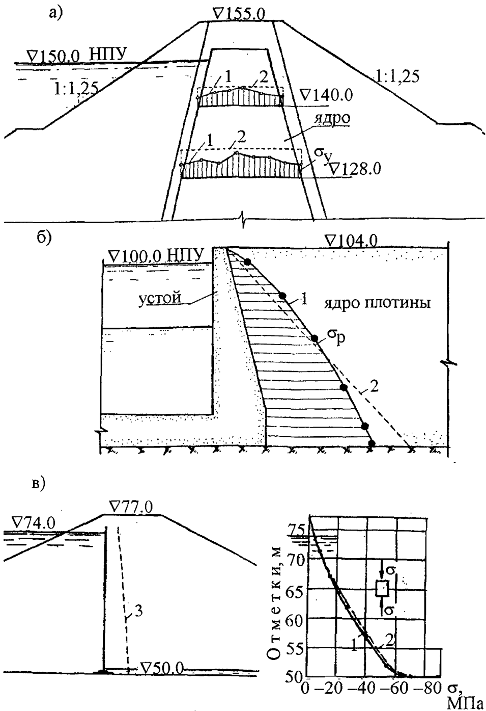
Рис.3.10. Натурные и расчетные эпюры нормальных сжимающих напряжений:
