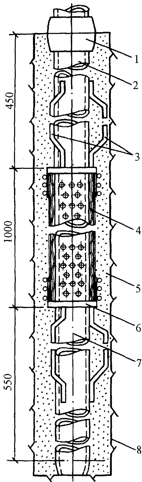
Рис.П1.11. Типовая конструкция водоприемника опускаемого пьезометра:
