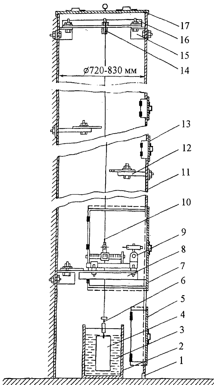
П.10. Измерительный узел прямого отвеса:
