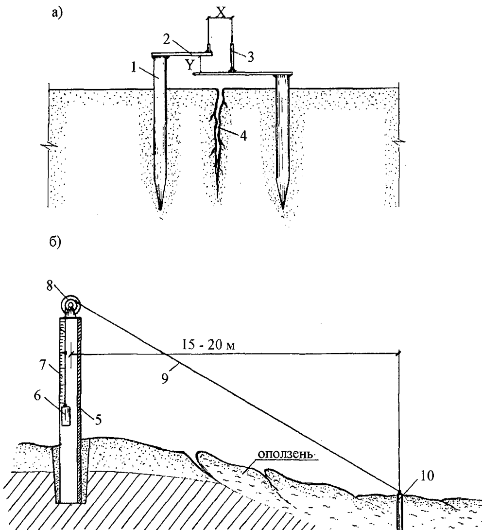
Рис.3.7. Схемы установки механического трещиномера на криогенной трещине (а); и шнуromера на откосе, подверженном солифлюкции (б):
