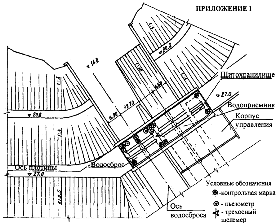
Схема размещения КИА на бетонных сооружениях Нижне-Терiberского гидроузла
