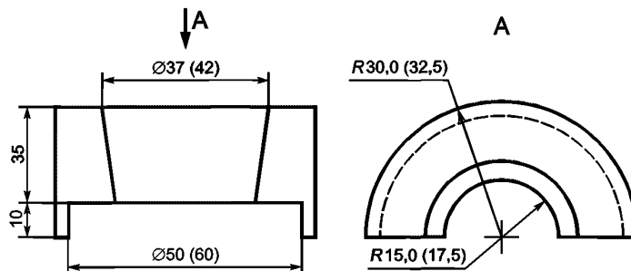
Рисунок 3 — Шаблон для круглой подставки
