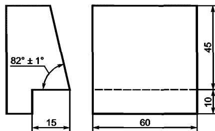
Рисунок 4 — Шаблон для прямоугольной подставки
