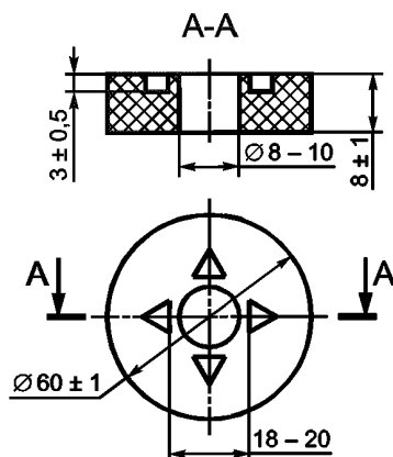
Рисунок А.1 — Подставка для вертикальной печи
