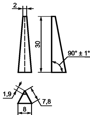
Рисунок 1 — Испытуемый конус
