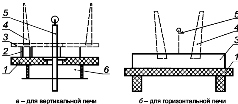
Рисунок А.1 — Подставка для вертикальной печи
