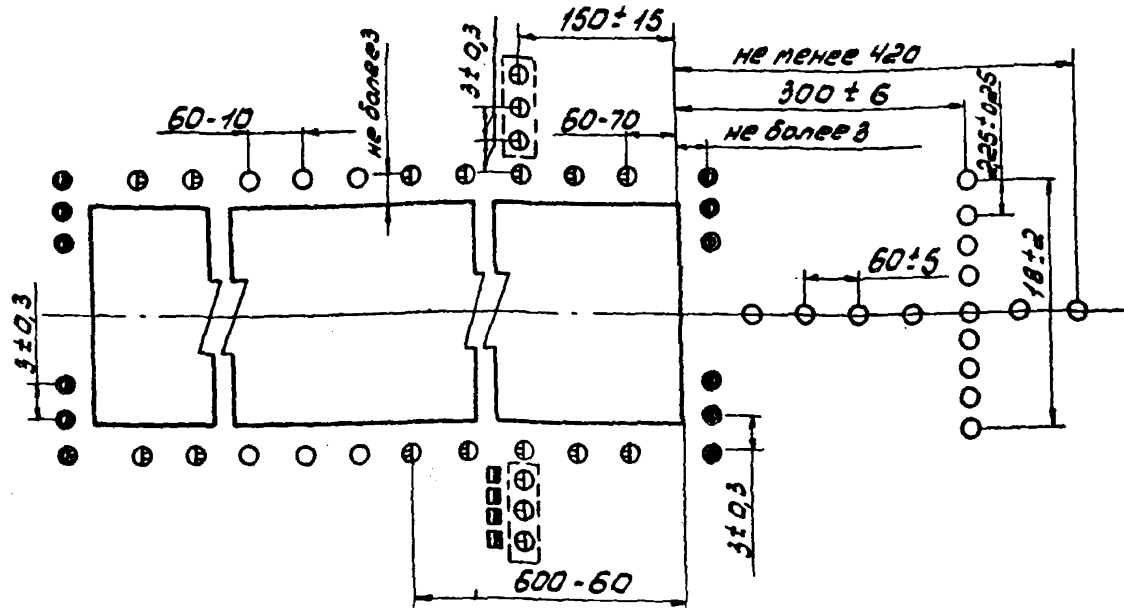
Рис. 1. Схема расположения светосигнального оборудования системы ОМИ для полетов по ЛВЛ: ○ - огонь приближения и светового горизонта; ● - входной ограничительный огонь зеленый-красный; ⊖ - посадочный огонь ВПП белый-желтый; ⊕ - огонь знака приземления белый; □ - глиссадный огонь
