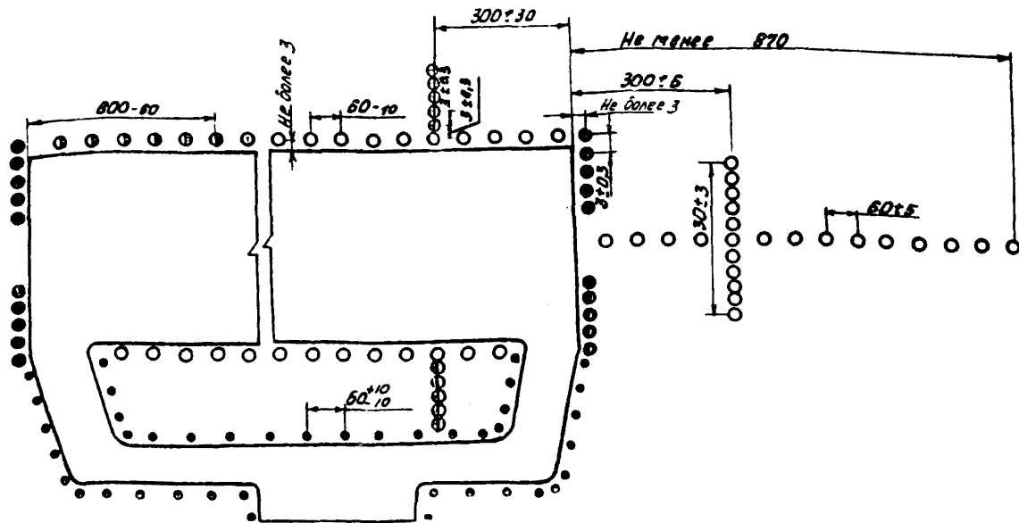
Рис. 2. Схема расположения светосигнального оборудования системы ОМИ для полетов по ПШ: ○ - огонь приближения, светового горизонта и посадочный ВПП белый; ⊕ - посадочный огонь ВПП на последних 600 м желтый; ⊙ - входной ограничительный огонь: зеленый - красный; ⊕ - огонь знака приземления белый; ● - рулежный огонь синий; ● - огра- ничительный огонь красный
