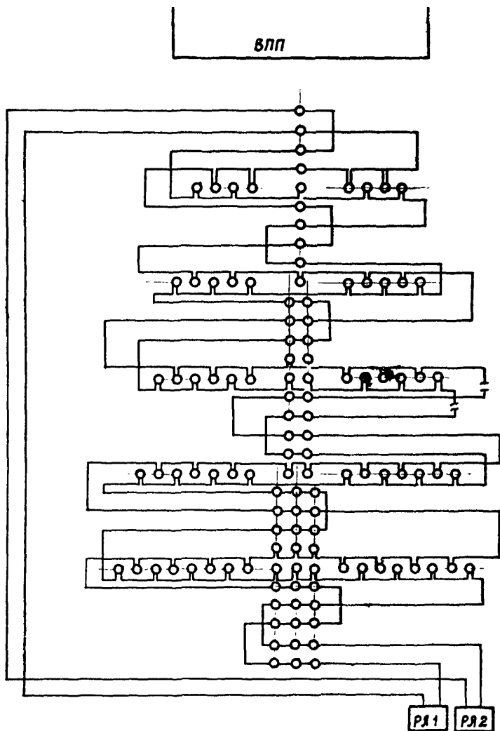
Рис. 15. Схема электропитания прожекторных огней приближения и световых горизонтов систем ОВН-1, ОВН-2 со световыми горизонтами
