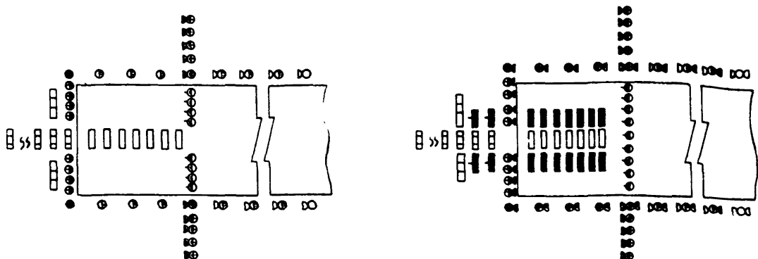
Рис. 10. Расположение светосигнального оборудования систем ОВИ при смещенном пороге:
