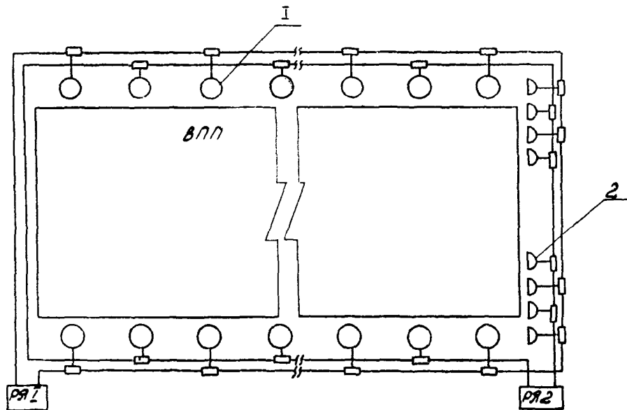
Рис. 23. Схема электропитания посадочных огней линзового типа и ограничительных огней прожекторного типа систем ОВИ-2 и ОВИ-3: 1 - линзовый огонь ВПП высокой интенсивности; 2 - прожекторный огонь ограничительный
