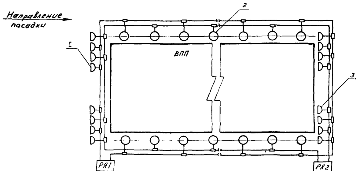
Рис. 22. Схема электропитания посадочных огней линзового типа, входных и ограничительных огней прожекторного типа систем ОВИ-I: 1 - прожекторный огонь входной; 2 - линзовый огонь ВПП высокой интенсивности; 3 - прожекторный огонь ограничительный
