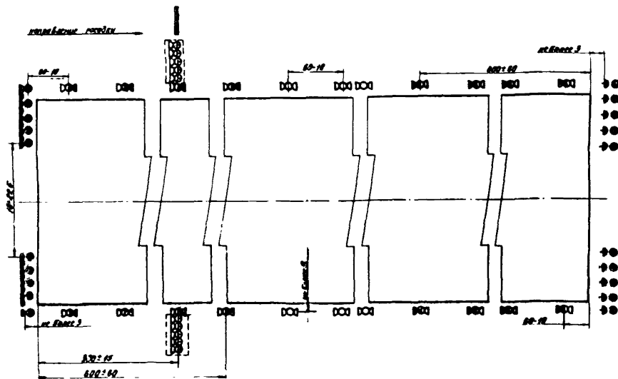
Рис. 5. Схема расположения огней на ВПП с одного направления посадки системы точного захода на посадку по категории I (ОВМ-I): ○ - посадочные огни кругового обзора белые; ● - входные огни прожекторные зеленые; ⊙ - входные-ограничительные огни кругового обзора зеленые-красные; ⊕ - посадочные огни ВПП знака приземления прожекторные белые; ⊖ - посадочные огни ВПП прожекторные желтые; ⊗ - ограничительные огни прожекторные красные; ⊕ - огни знака приземления кругового обзора белые с заглушкой; ⊔ - глиссадные огни; ⊕ - посадочные огни ВПП кругового обзора белые-желтые
