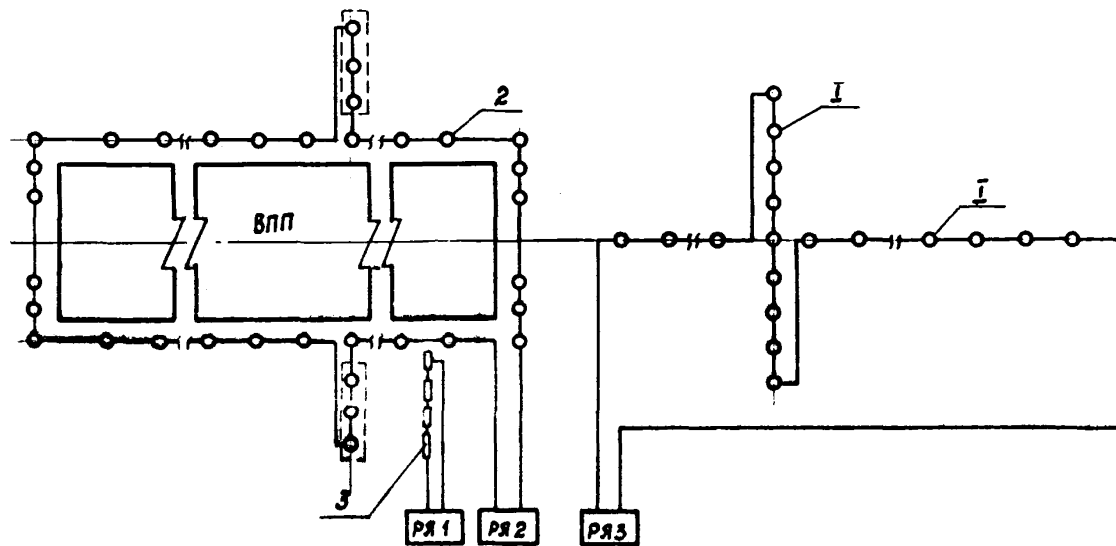
Рис. 24. Схемы электропитания огней в светосигнальных системах ОММ: I - огни приближения и светового горизонта кругового обзора; 2 - огни ВПП; 3 - галссадные огни
