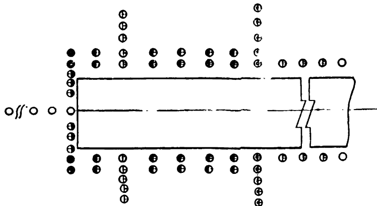
Рис. 9. Расположение светосигнального оборудования систем ОМ при смещенном пороге: ⊕ - посадочный огонь ВПП, огонь светового горизонта белый-желтый; ⊗ - посадочный огонь красный-желтый; ⊖ - посадочный огонь красный (с половинной заглушкой); ⊙ - посадочный огонь красный; ⊕ - входной фланговый огонь зеленый (с половинной заглушкой); ⊗ - входной посадочный огонь зеленый-желтый; ⊖ - огонь светового горизонта белый (с половинной заглушкой); ⊙ - ограничительный огонь красный (с половинной заглушкой); ○ - огонь приближения и посадочный ВПП белый.
