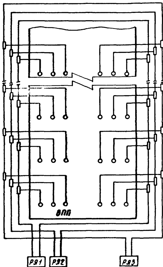
Рис. 14. Схема электропитания огневой зоны приземления систем ОБИ-2 со световыми горизонтами
