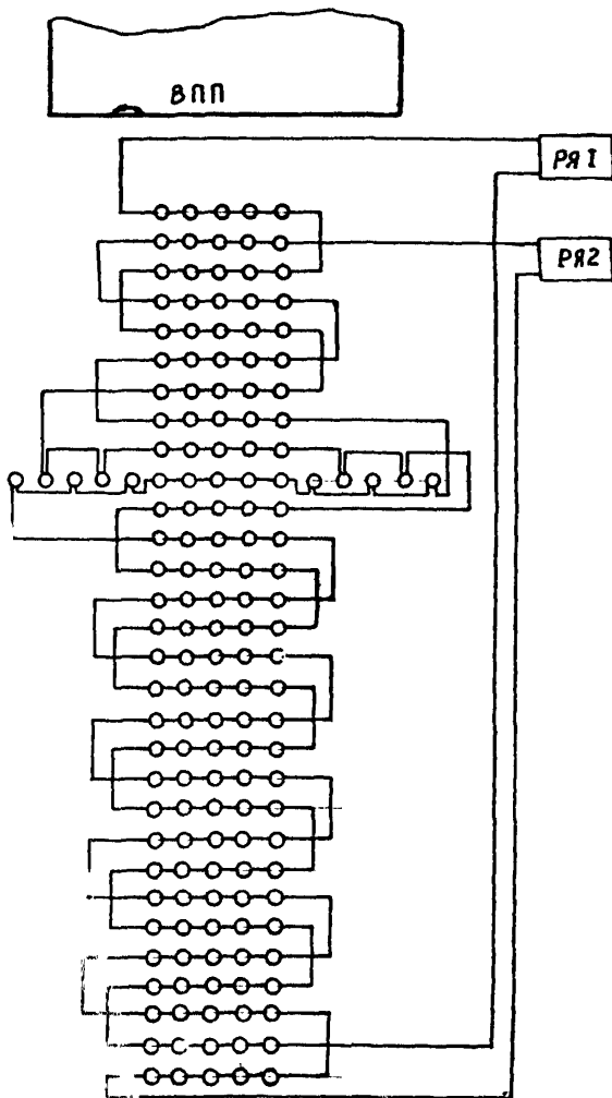
Рис. 16. Схема электропитания прожекторных огней приближения и светового горизонта систем ОБИ-1, ОБИ-2 и ОБИ-3 с огнями приближения по центральному ряду
