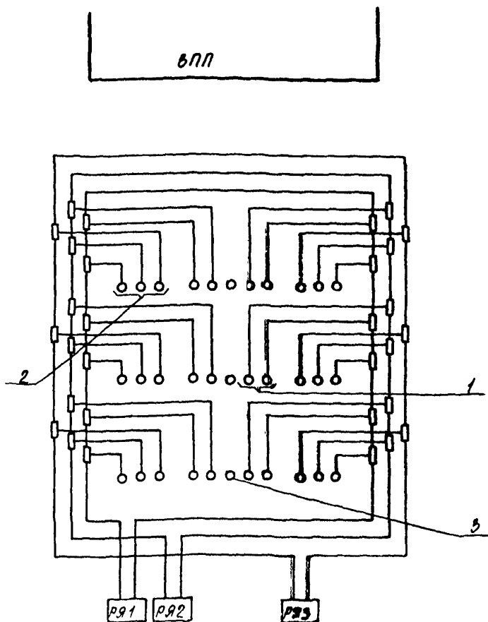
Рис. 13. Схема электропитания прожекторных огней центрального ряда и боковых огней на КПБ систем ОБИ-2 со световыми горизонтами: 1 - огни КПБ центрального ряда прожекторные; 2 - огни КПБ бокового ряда прожекторные; 3 - осевые огни КПБ прожекторные
