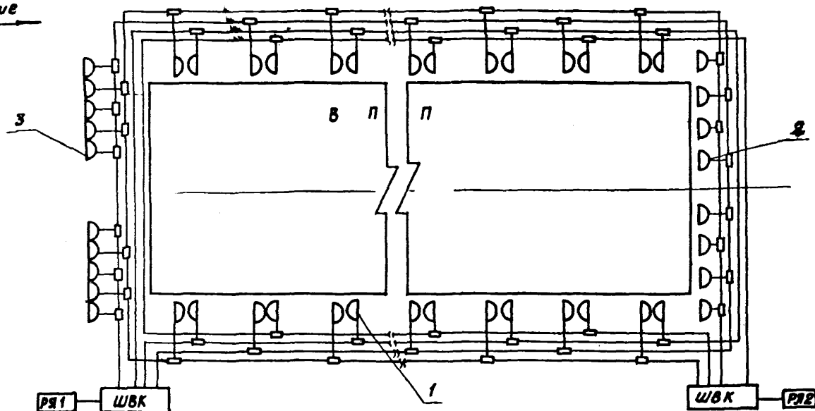
Рис. 19. Схема электропитания посадочных, входных и ограничительных огней прожекторного типа систем ОБИ-1: 1 - посадочный огонь; 2 - ограничительный огонь; 3 - входной огонь
