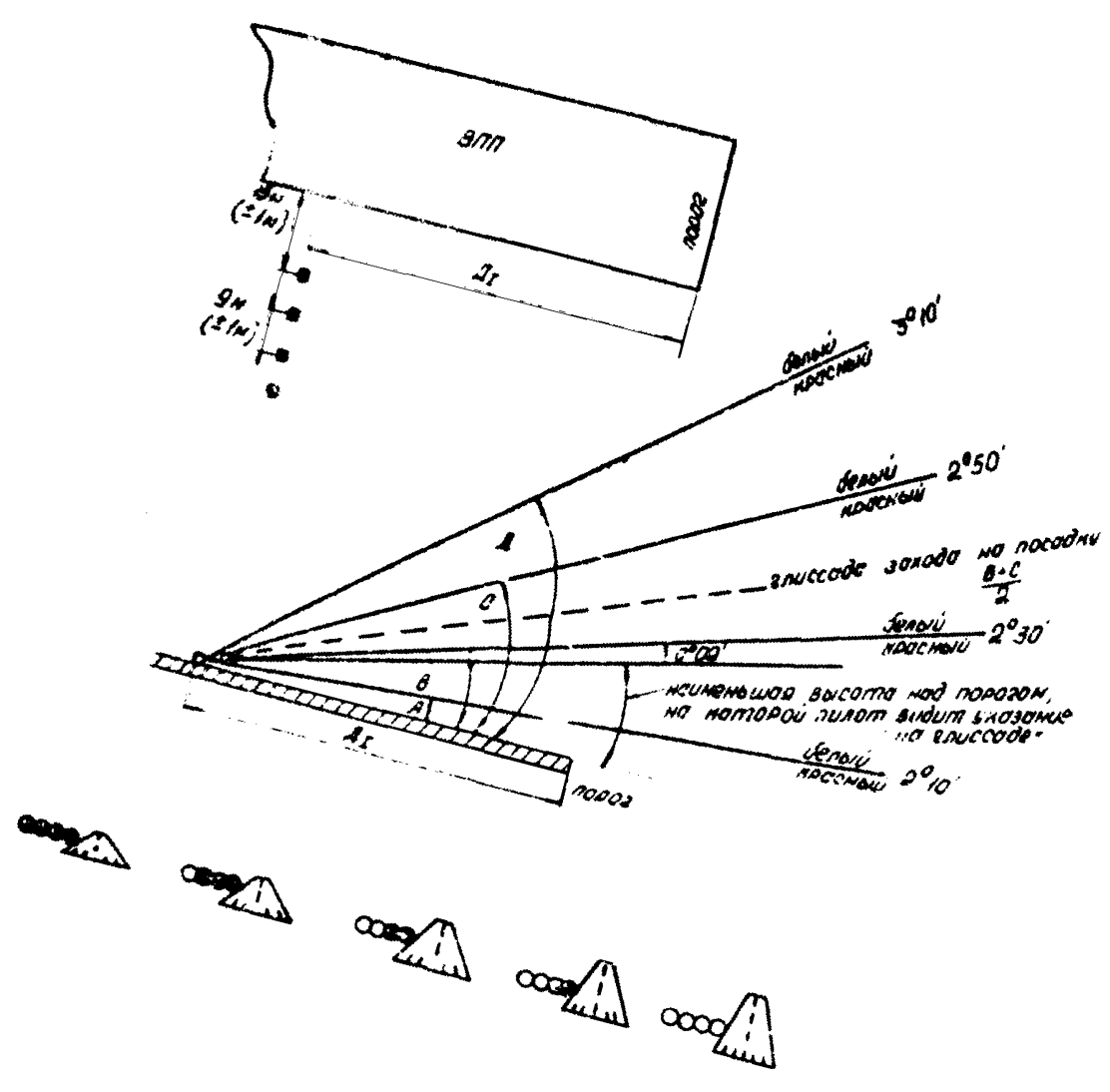
Схема расположения огней системы PARU и распределе- ние углов возвышения огней (угол захода на посадку 2°40')
