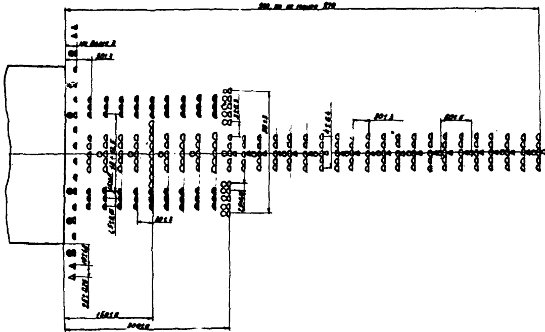
Рис. 6. Схема расположения огней приближения и входных огней систем точного захода на посадку по категориям II и III (ОВИ-2, ОВИ-3): ● - боковые огни КПБ прожекторные красные; ○ - огни приближения и светового горизонта прожекторные белые; ○ - огни приближения и светового горизонта кругового обзора белые; ▽ - огни приближения импульсные белые; ▽ - входные огни импульсные зеленые.
