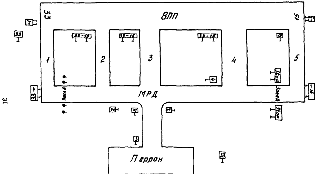
Рис. II. Размещение неуправляемых световых указателей: 33 - неуправляемый световой указатель
