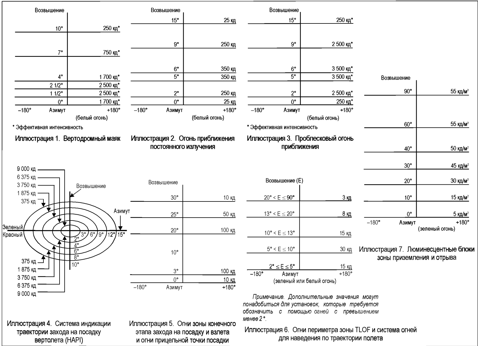
Рис. 5-11. Диаграммы изокандели
