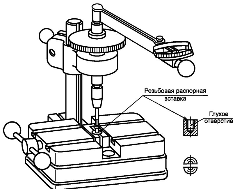
Рисунок 1 — Пример устройства для испытания на кручение
