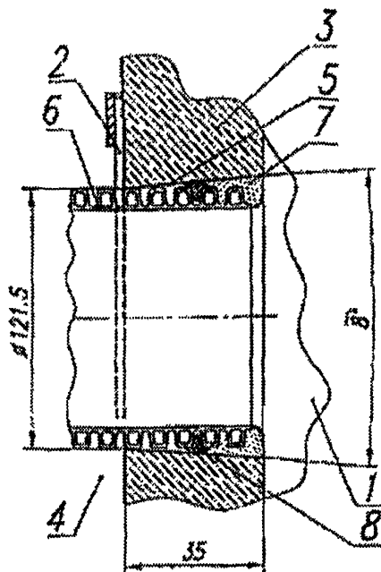
Рис.6. Схема ввода ПТТ в железобетонные телефонные колодцы конструкции ЗАО «Связьстройдеталь» 1-внутренняя полость колодца, 2- фиксатор трубы, 3- стенка колодца, 4- внешнее пространство, 5- конусное отверстие в стене, 6- ПТТ, 7- цементно-песчаная заделка, 8- резиновое уплотнение
