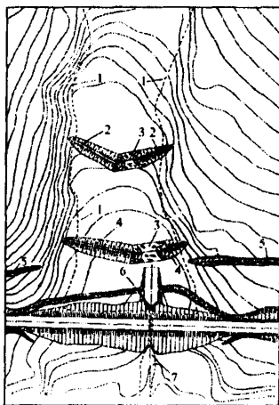
Рис. 36. Противоналедные валы:
