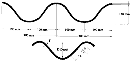
Рис.А.4. Профиль гофрированного листа Толщина листа 3,5-7,1 мм, углы изгиба гофра 49,75-50,43^\circ Прямая вставка 110,78 - 106,15 мм
