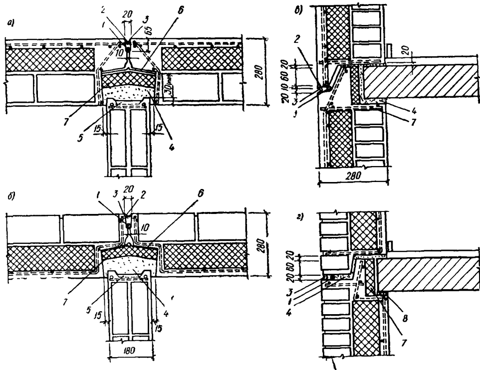
Рис. 64. Стыки панелей
