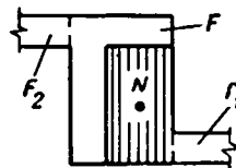
Рис. 19. Расчетная сжатая часть сложного сечения при косом внецентренном сжатии. Площади F_1 и F_2 в расчете не учитываются
