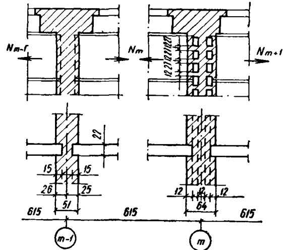
Рис. 117. К расчету кладки поперечных стен в местах заделки плит перекрытий
