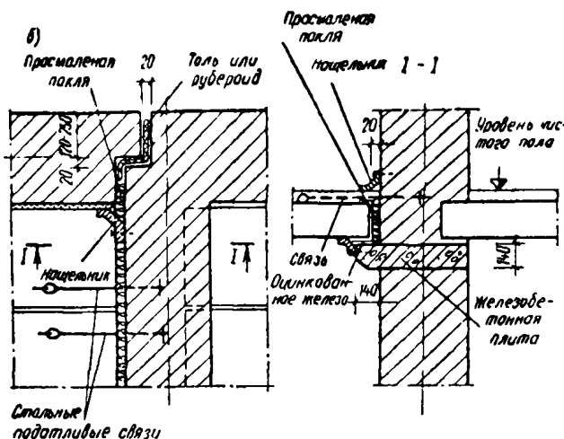
Рис. 83. Температурные швы в зданиях с поперечными несущими стенами
