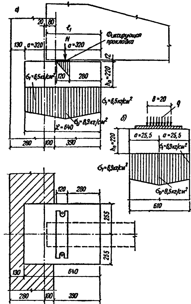
Рис. 28 а — Схема узла опирания балки на стену с пилястрой и распределение напряжений в кладке под опорной плитой в направлении оси балки б — Схема узла опирания балки на стену с пилястрой и распределение напряжений в кладке под опорной плитой в поперечном направлении
