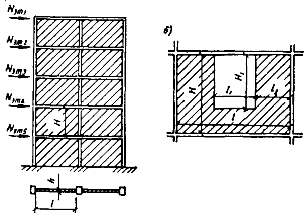
Рис. 39. К расчету каркасных стен
