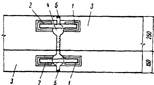
Рис. 67. Стык перемышечных (поясных) блоков 1 — закладные детали и связи; 2 — сварной шов; 3 — перемышечные (поясные) блоки; 4 — раствор; 5 — расшивка раствором
