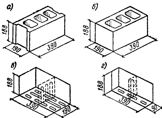
Рис. 3. Бетонные пустотелые камни
