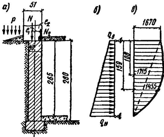
Рис. 96 К примеру 16. Расчет стены подвала
