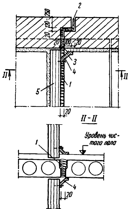
Рис. 85. Температурные швы в зданиях с продольными несущими стенами у поперечной перегородки 1 — просмоленная покля; 2 — толь или рубероид с утеплителем; 3 — расшивка шва; 4 — нащельник; 5 — перегородка
