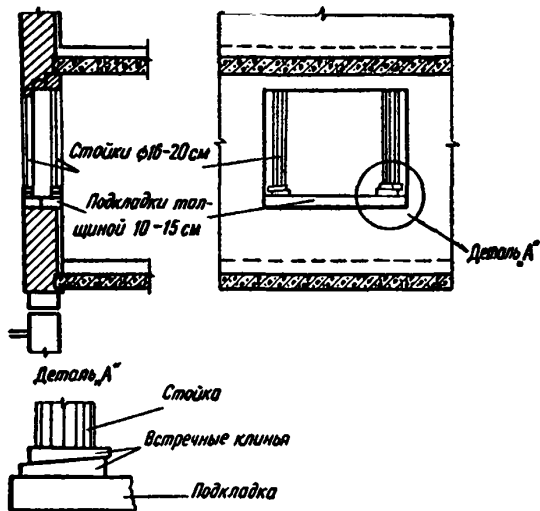
Рис. 101. Усиление проstenка временными деревянными стойками
