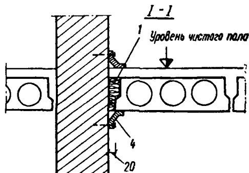
Рис. 84. Температурные швы в зданиях с продольными несущими стенами
