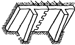
Рис. 11. Растяжение кладки при изгибе по перевязанному сечению
