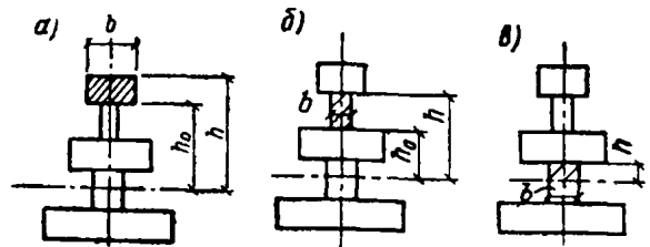
Рис. 106. Размеры к расчетным формулам
