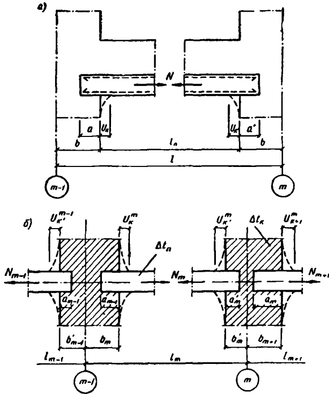
Рис. 113. Расчетные схемы работы кладки с армированными элементами
