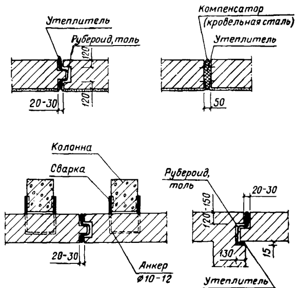
Рис. 86. Температурные швы в стенах промышленных зданий
