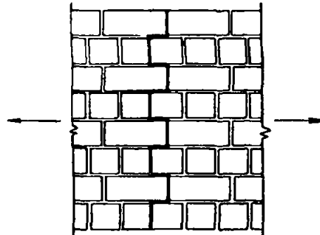
Рис. 10. Растяжение кладки по перевязанному сечению
