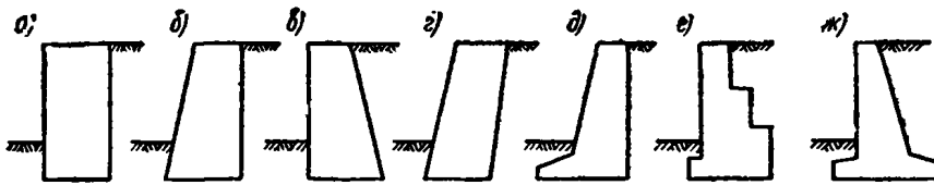
Рис. 88. Подпорные стены разных профилей
