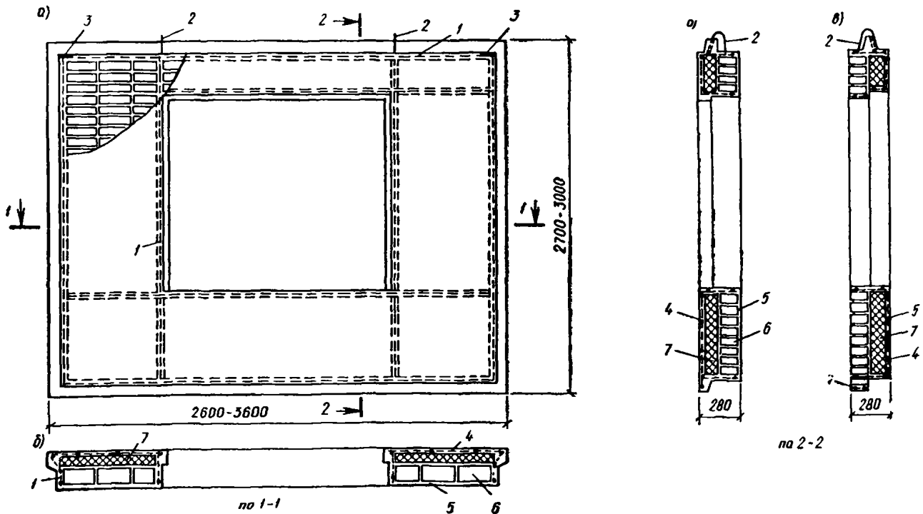
Рис. 62. Двухслойная кирпичная панель наружной стены
