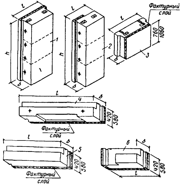
Рис. 4. Основные типы крупных блоков наружных стен для жилых зданий
