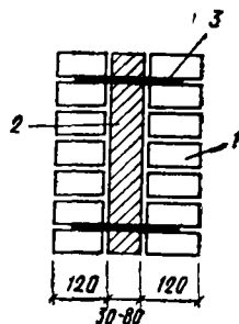
Рис. 54. Стена типа VI с теплоизоляцией внутри кладки
