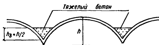
Рис. 95. Своды комплексной конструкции
