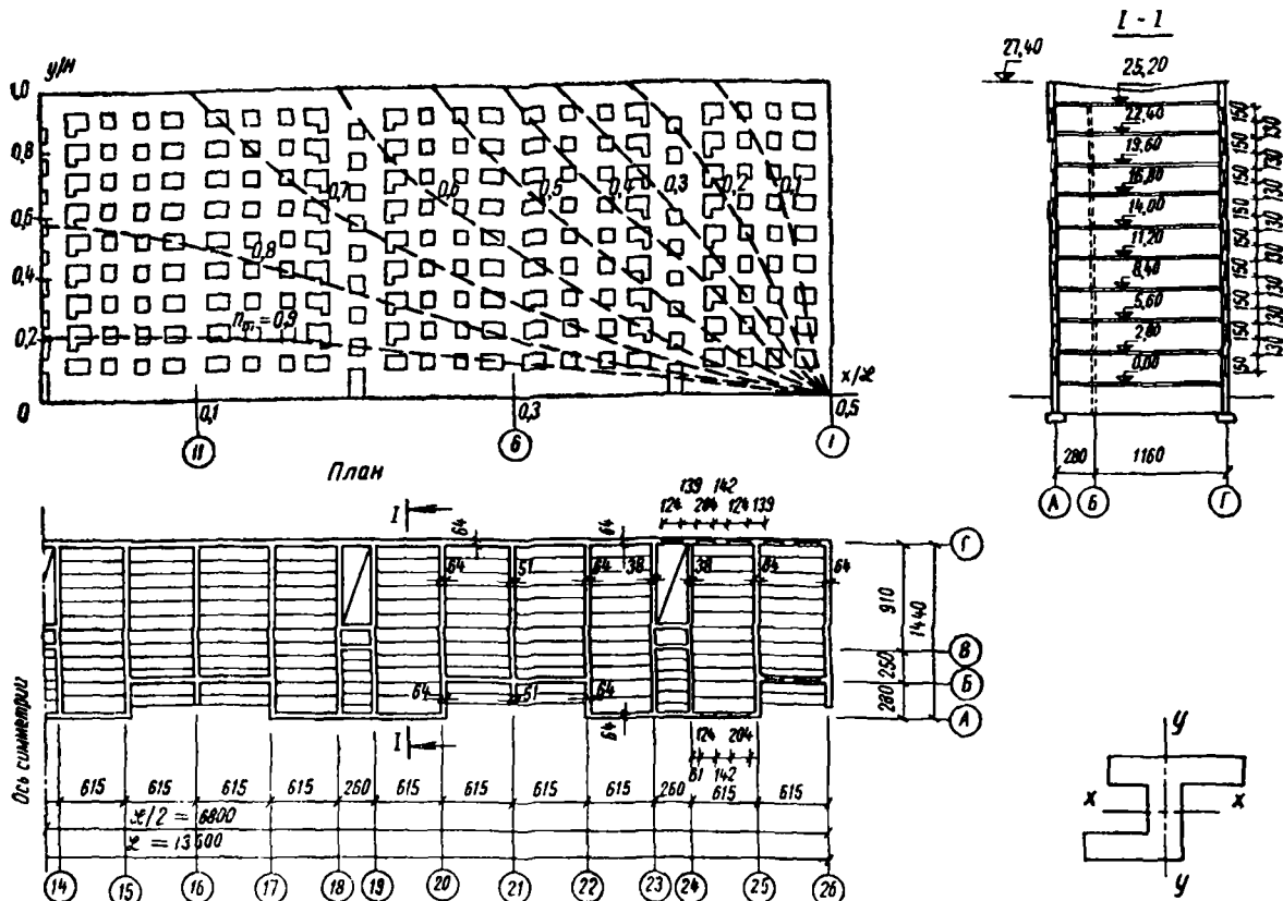
Рис. 115. План, фасад и разрез 9-этажного жилого дома длиной 136 м без температурных швов
