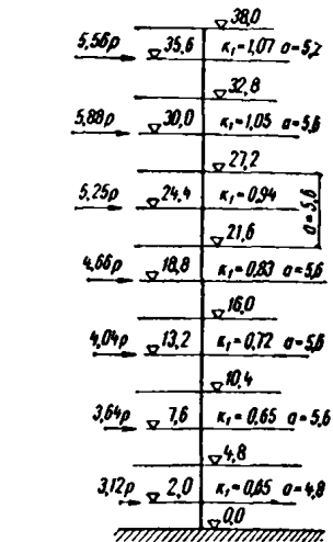
Рис. 44. Схема нагрузок
