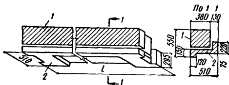
Рис. 6. Перемычковый кирпичный блок
