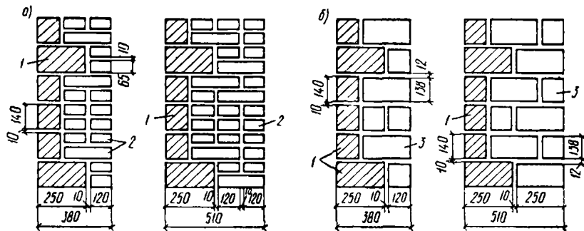
Рис. 70. Кладка типа XIIa из кирпича или керамических камней совместно с лицевыми керамическими камнями
