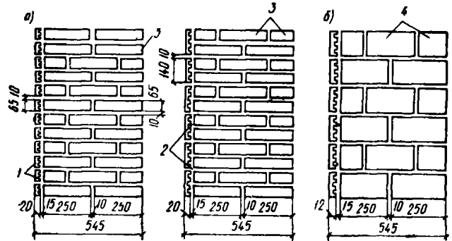
Рис. 74. Облицовка кладки прислонными керамическими плитками с креплением на растворе
