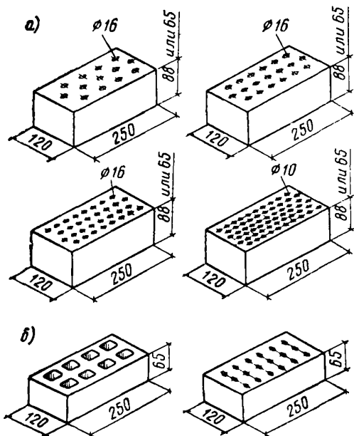
Рис. 1. Пустотелый кирпич
