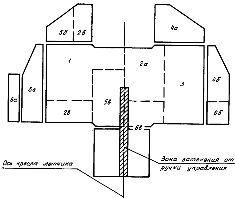
Зоны приборной доски летчика учебно-тренировочного самолета
