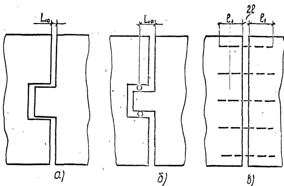
Рис. I. I. Схематическое изображение узлов соединения секций в зоне температурного шва. (план) а, б) - зубцы, в) шпирями.
