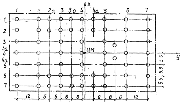
Рис. 3.2. План свайного поля нефтепровода.
