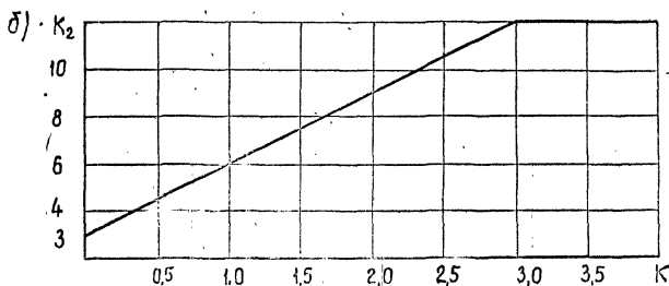
Рис. I. 2. Графики коэффициентов K_1 и K_2 .
