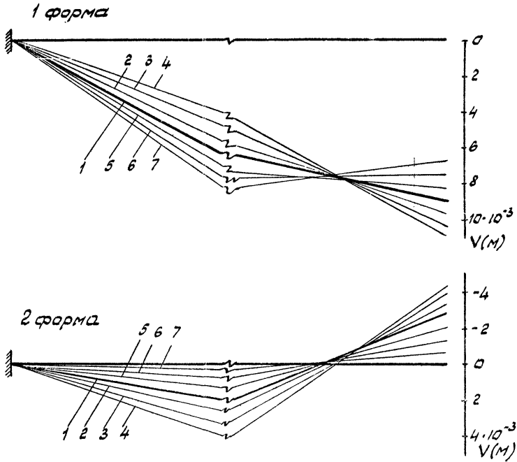
Рис. 3.6 формы деформации шпруса при сейсмических колебаниях для различных значений e_{2y} : 1) e_{2y} = 0 , 2) e_{2y} = -1\%L , 3) e_{2y} = -2\%L , 4) e_{2y} = -3\%L , 5) e_{2y} = 1\%L , 6) e_{2y} = 2\%L , 7) e_{2y} = 3\%L .
