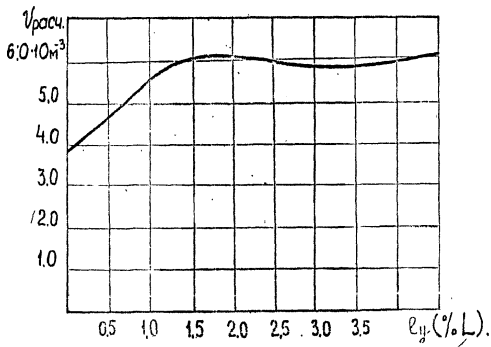
Рис. 3.3. График V_{расч}(v_y) .
