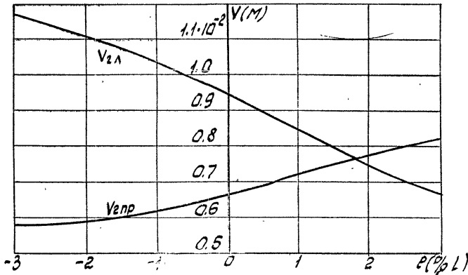
Рис. 3.7 График зависимости суммарных прогибов левого и правого концов второй секции от величины эксцентриситета e_{2y} .
