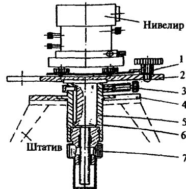
Рис. 1. Прецизионная нивелирная подставка
