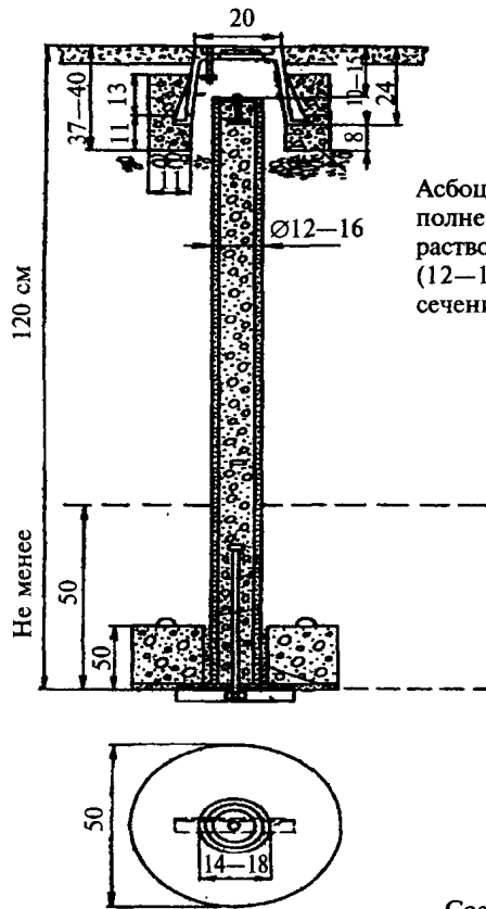
Бетонный якорь Ø50 см
