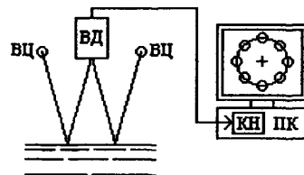
Рис.2. Схема видеоуровнемера
