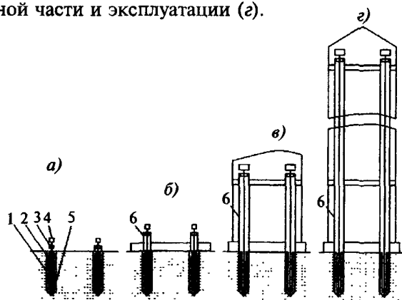
Рис. 3. Схема использования обратного отвеса
