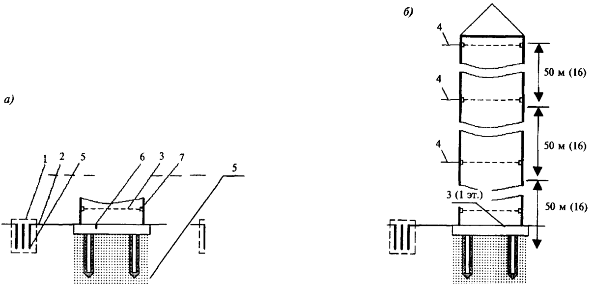
Рис. 7.1. Типовая схема высотной основы для наблюдения за деформациями
