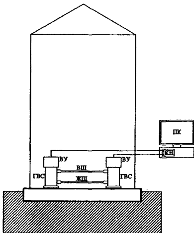
Рис.1. Схема видеогидростатической системы
