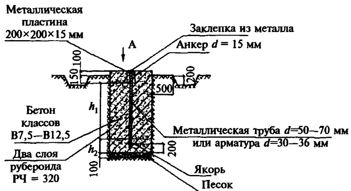
Знак закрепления оси
