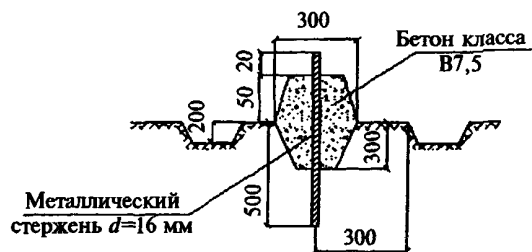
Знак закрепления временных осей и точек внутренней разбивочной основы
