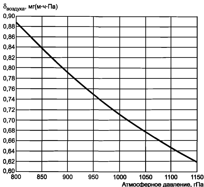
Рисунок 1 — Паропрооницаемость воздуха при 23 °C
