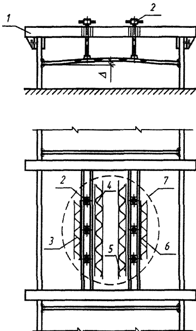
1 – рама; 2 – винтовой прижим; 3, 6 – полосы нагрева первого этапа правки; 4, 5 – то же второго этапа; 7 – граница «хлопуна»
