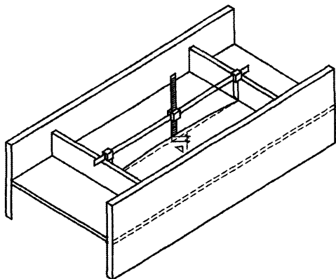
Рисунок 5.5 – Измерение выпучивания («хлопуна») в замкнутом контуре
