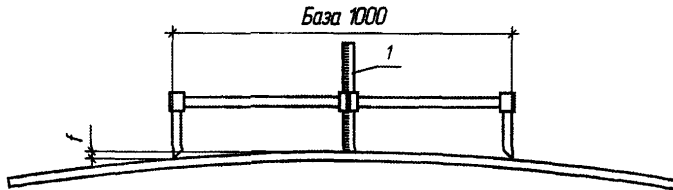
Рисунок 5.1 – Измерение выпучивания и волнистости листа
