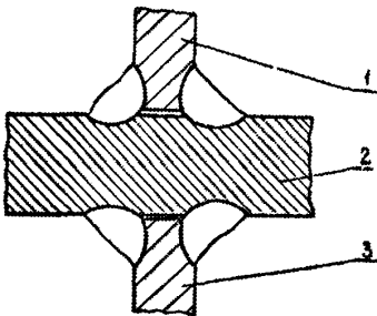
Рисунок А.2.5 – Прикрепление к элементу втавр с двух сторон деталей четырьмя сближенными швами
