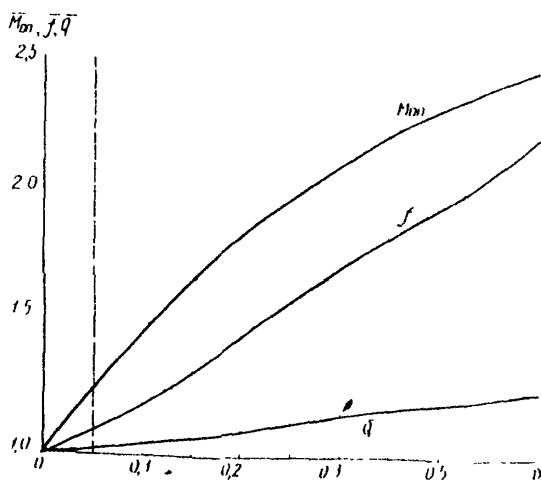
Рис. 29. Графики для определения \overline{M}_{on} , \overline{F} и \overline{q} при расчете двухленточных переходов
