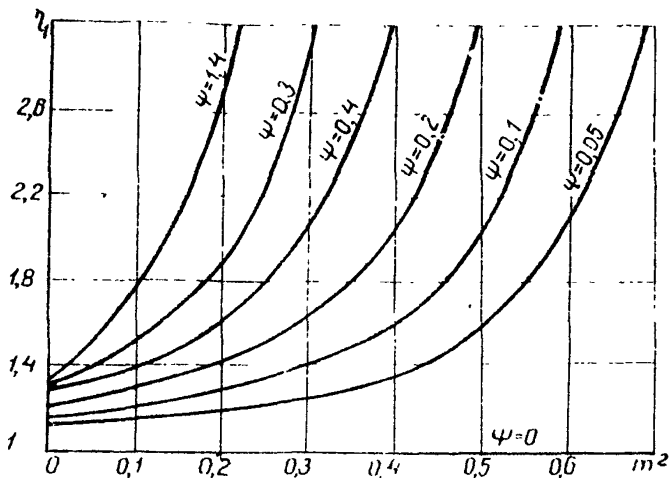
Рис.24. График зависимости безразмерного параметра \eta_1 от m^2 и \psi
