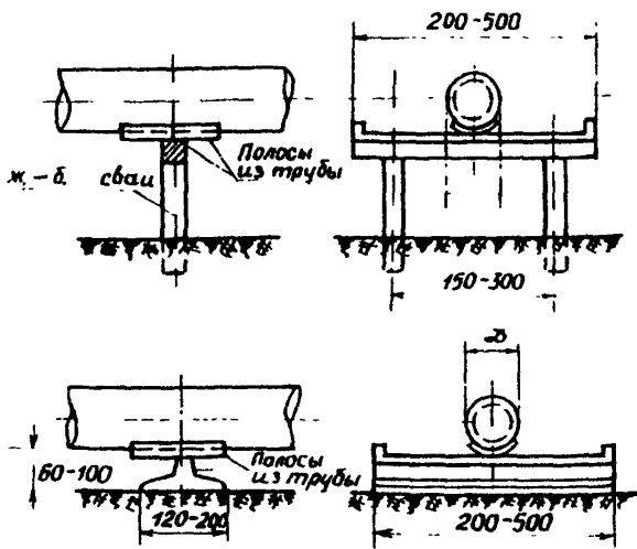
Рис.15. Схемы промежуточных опор надземных переходов
