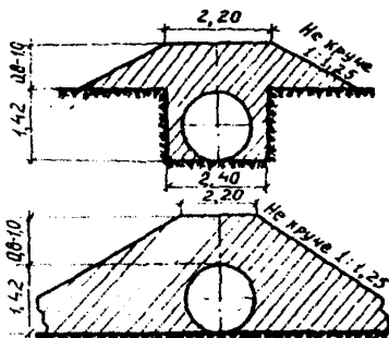
Рис.2. Укладка трубопровода: а-полузаглубленная; б-наземная
