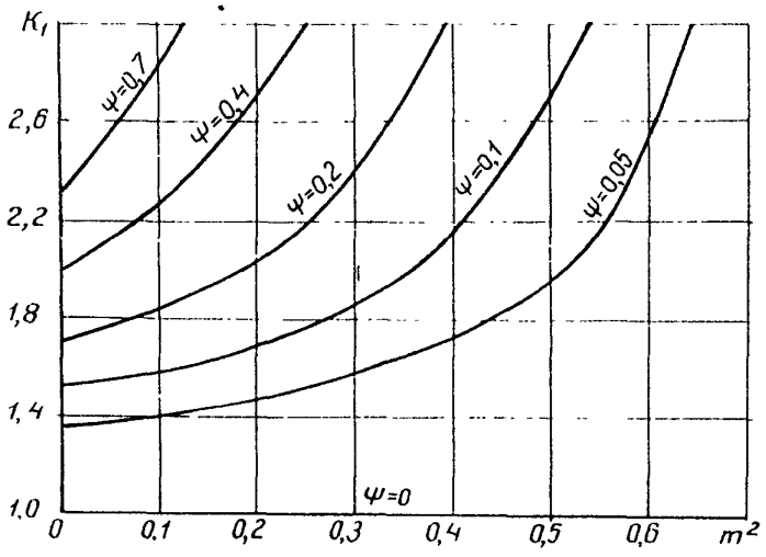
Рис.26. График зависимости безразмерного параметра K_1 от m^2 и \psi
