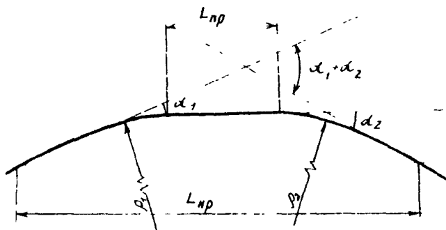
Рис.18. Расчетная схема трубопровода, когда на длине волны выпучивания имеется две кривые с прямолинейной вставкой между ними
