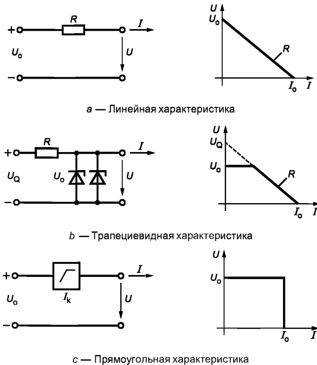
Рисунок С.1 — Характеристики эквивалентных цепей и выходов резистивных цепей
