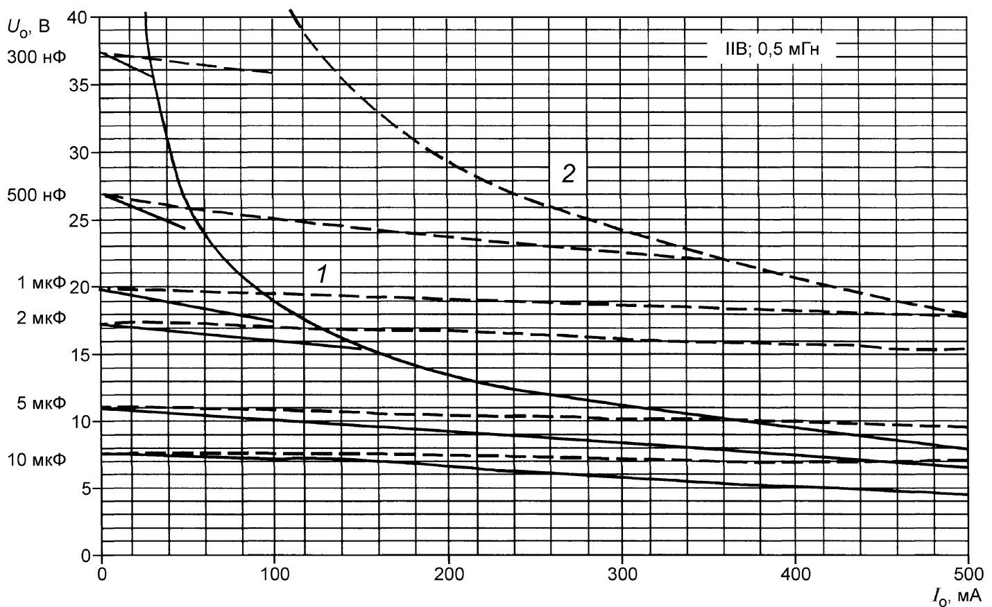
Рисунок С.8а — Диаграмма для значения 0,15 мГн (продолжение)
