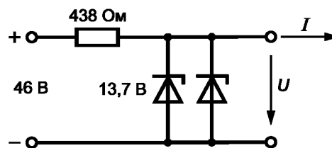
б — эквивалентная цепь
