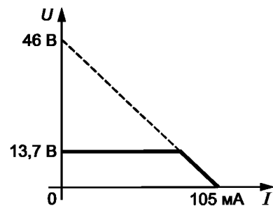
а — выходные характеристики
