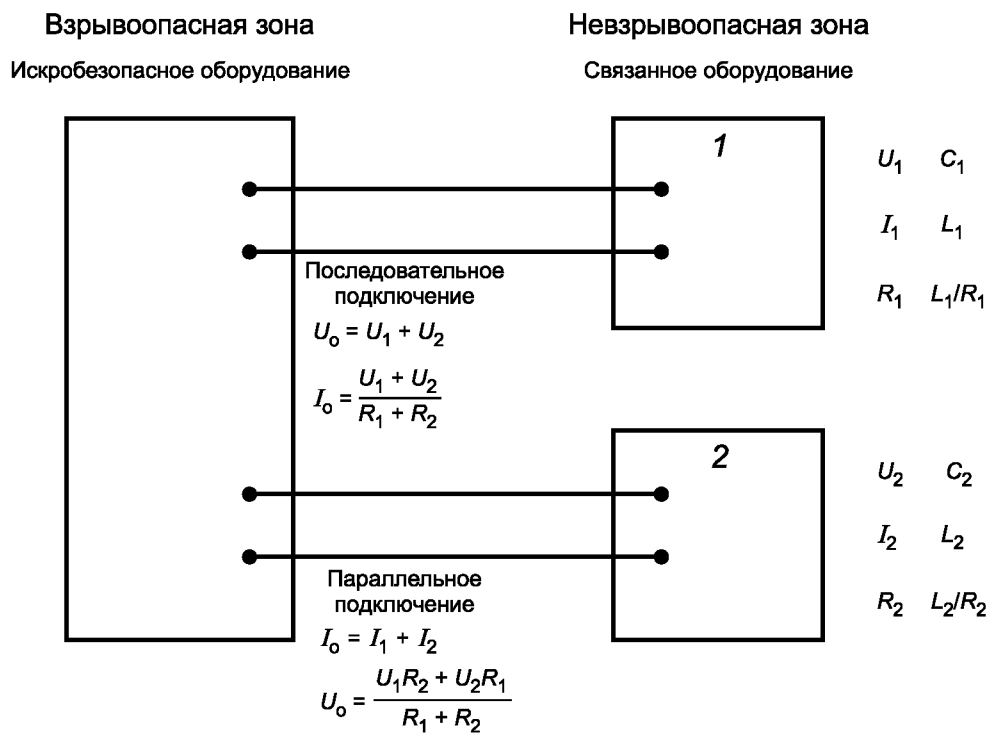
Рисунок В.3 — Источники питания, подключенные произвольно
