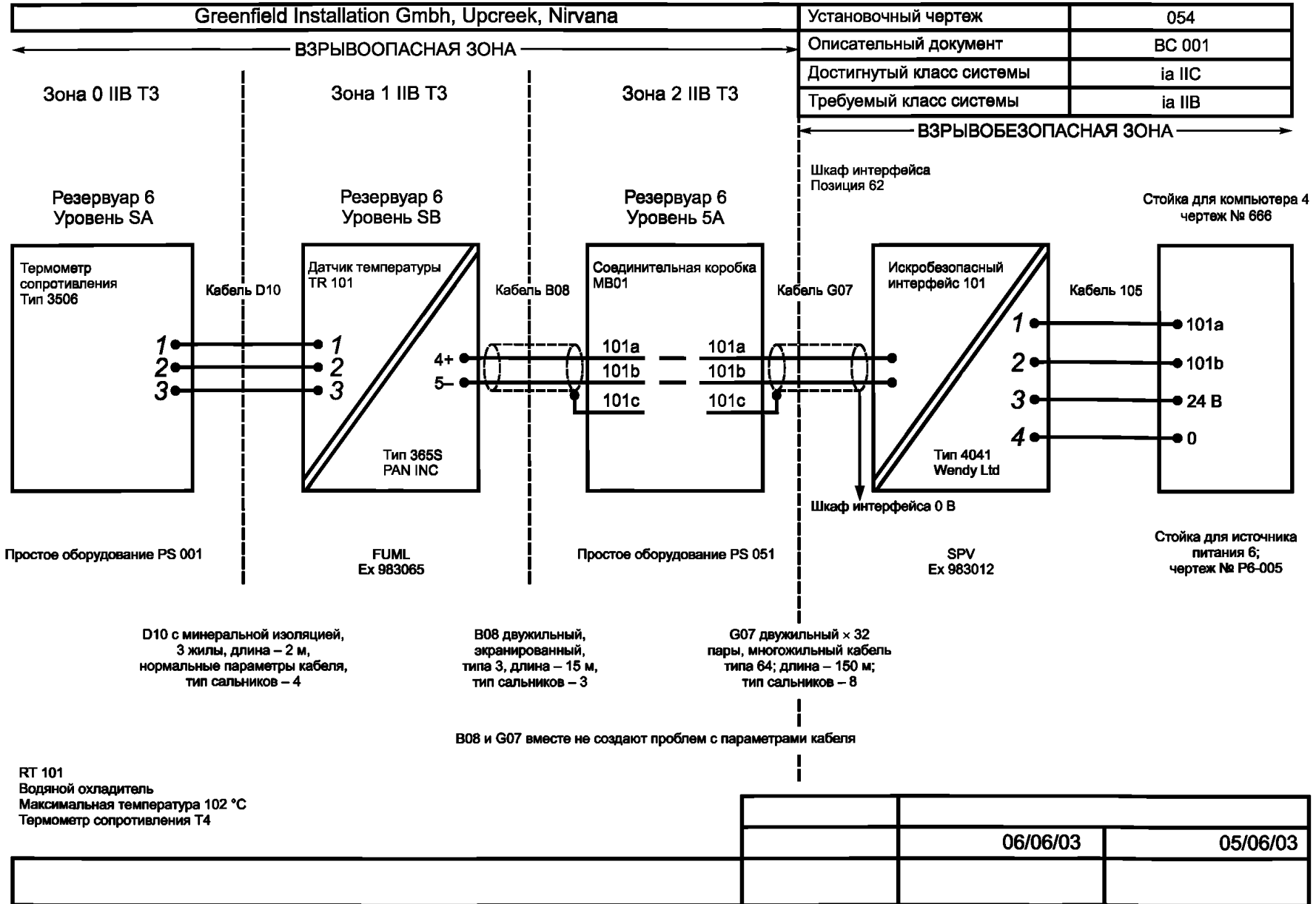
Рисунок Е.2 — Типовая схема соединений искробезопасной системы
