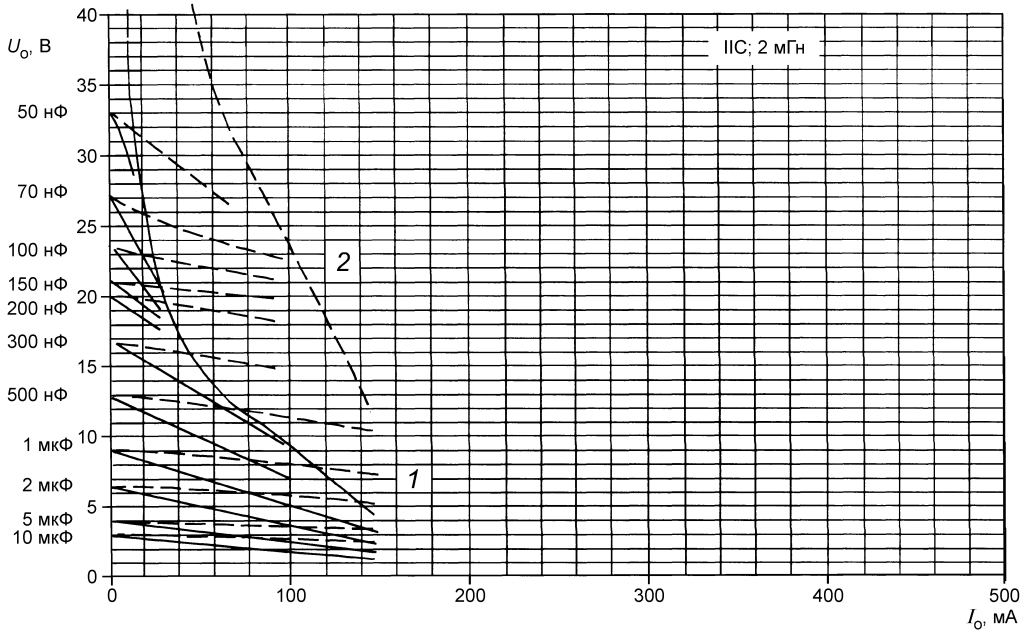
Рисунок С.7d — Диаграмма для значения 2 мГн (продолжение)
