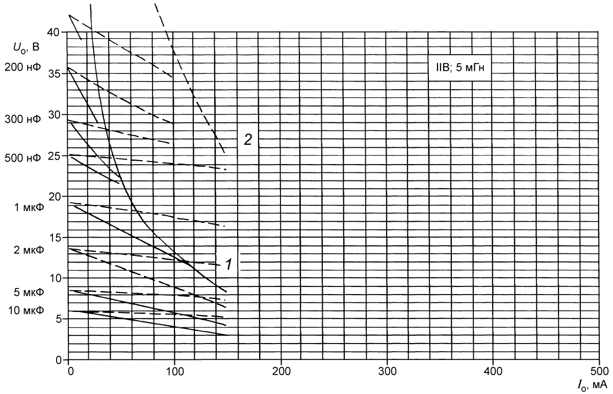
Рисунок С.8е — Диаграмма для значения 5 мГн (продолжение)
