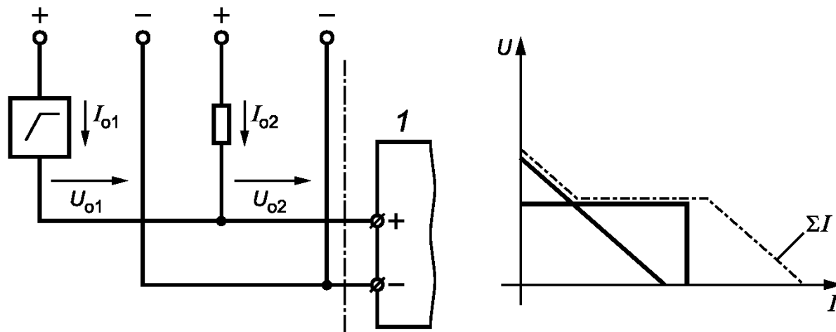
c — Параллельное подключение со сложением значений тока
