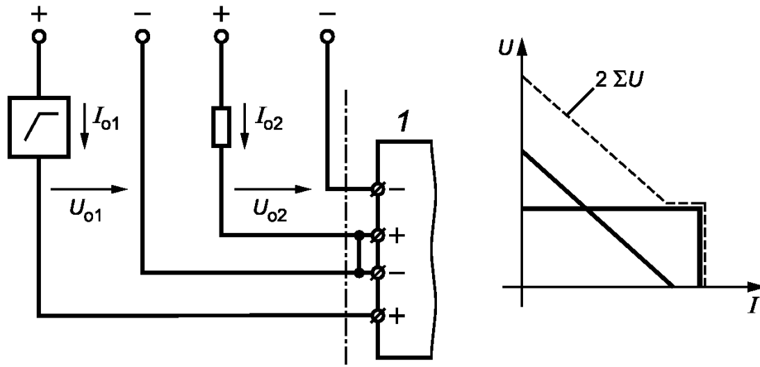
b — Последовательное подключение со сложением значений напряжения и возможным сложением значений тока
