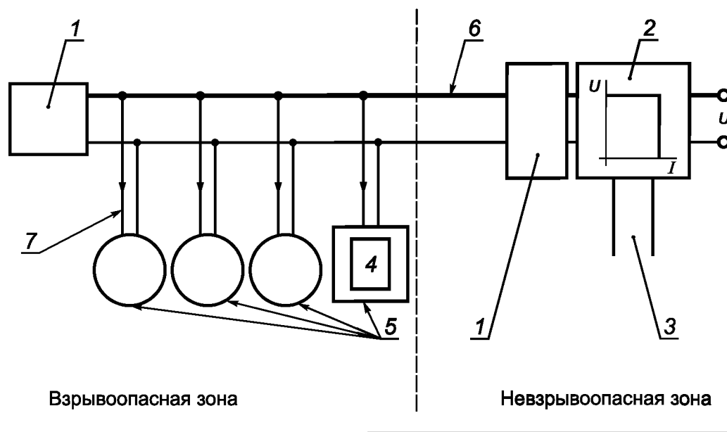
1 — оконечное устройство; 2 — источник питания; 3 — данные; 4 — ручной терминал; 5 — полевые устройства; 6 — магистральный кабель; 7 — ответвительный кабель
