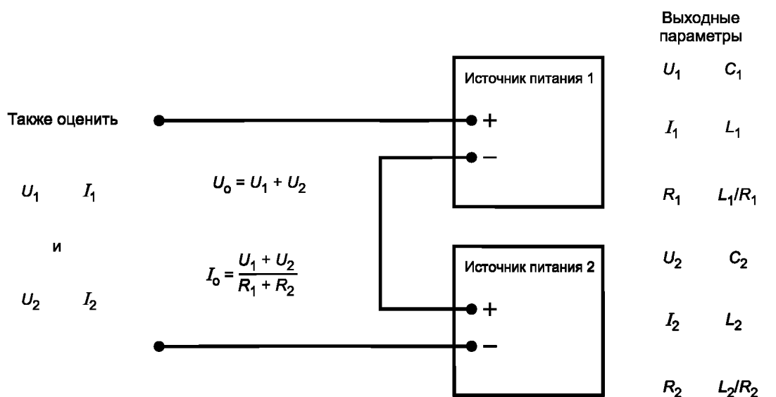
Рисунок В.1 — Источники питания, подключенные последовательно
