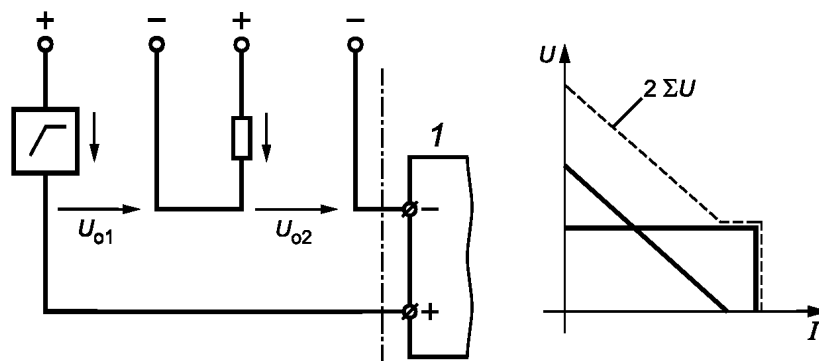
а — Последовательное подключение со сложением значений напряжения
