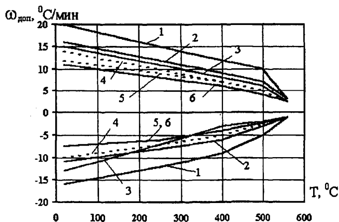
Рис.1. Допустимые скорости \omega_{\text{доп}} прогрева и расхолаживания паропроводов свежего пара (1 - 194×36 мм; 2 - 245×45 мм; 3 - 219×32 мм; 4 - 219×52 мм; 5 - 325×60 мм; 6 - 275×62,5 мм).
