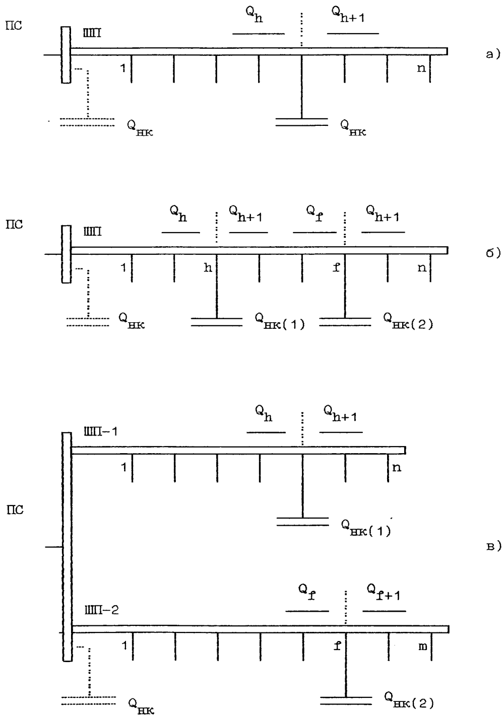
Рис. 2-6. Схема подключения БНК к магистральным шинопроводам: а - одна БНК; б - две БНК; в - два магистральных шинопровода с установкой по одной БНК
