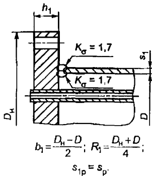
Рисунок 7 — решетка, приваренная втавр к обечайке кожуха
