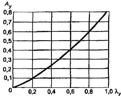
Рисунок 12 — Коэффициент для определения максимального прогиба трубы
