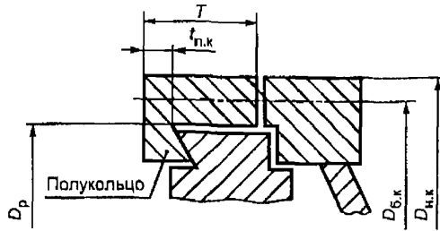
Рисунок 13 — Элементы плавающей головки
