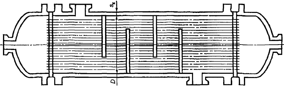
Рисунок 1 — Аппарат с неподвижными трубными решетками
