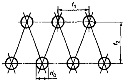
Рисунок Ж.2 — Расположение отверстий по вершинам треугольников
