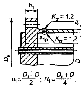
Рисунок 8 — решетка, приваренная встык к обечайке кожуха
