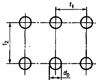
Рисунок Ж.1 — Расположение отверстий по вершинам прямоугольников
