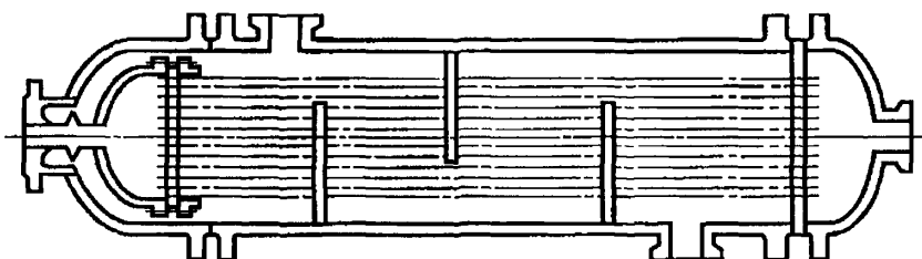
Рисунок 6 — Аппарат с компенсатором на плавающей головке
