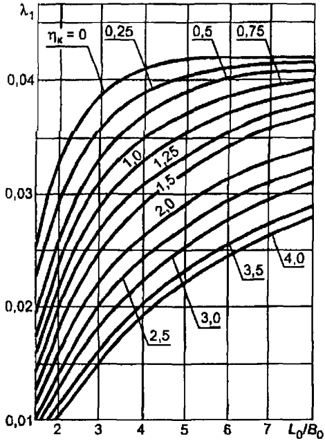
Рисунок И.1 — График коэффициента \lambda_1
