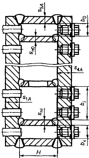
Рисунок 23 — Сварная камера с перегородками
