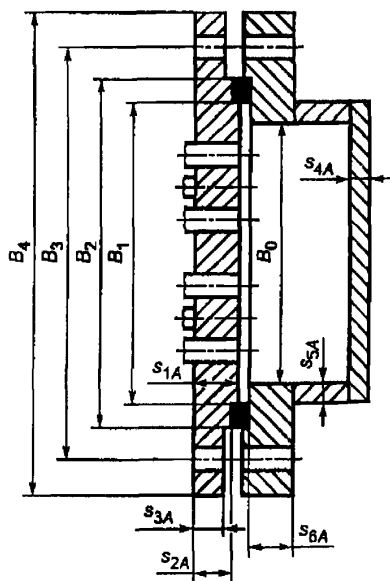
Рисунок 15 — Камера разъемной конструкции со сварной крышкой
