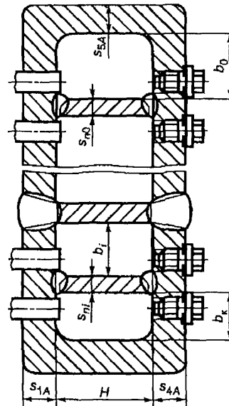
Рисунок 24 — Штампованная камера с перегородками
