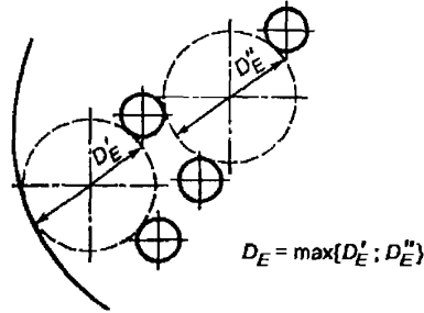
Рисунок 14 — Диаметр окружности, вписанной в максимальную беструбную площадь
