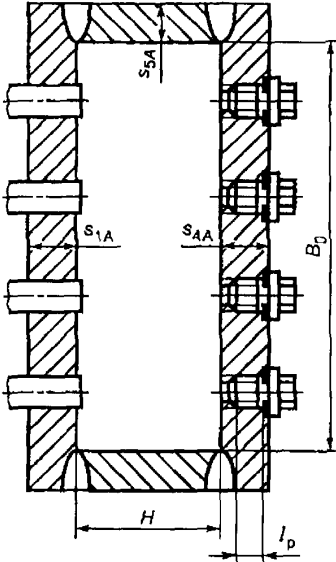
Рисунок 21 — Сварная камера без перегородок
