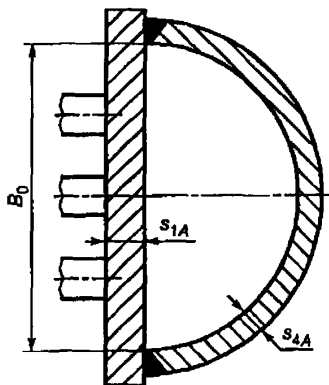
Рисунок 20 — Камера неразъемной конструкции с полуцилиндрической задней стенкой
