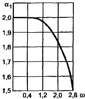
Рисунок И.3 — График коэффициента \alpha_1
