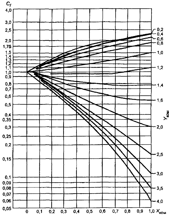
Рисунок 25 — Параметр жесткости компенсатора C_f
