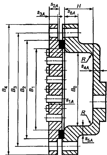
Рисунок 16 — Камера разъемной конструкции с литой крышкой
