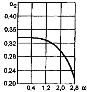
Рисунок И.4 — График коэффициента \alpha_2
