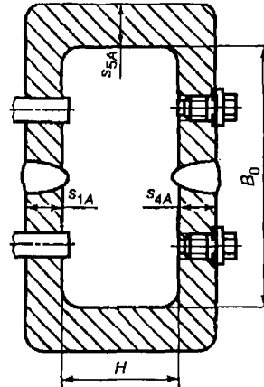
Рисунок 22 — Штампованная камера без перегородок
