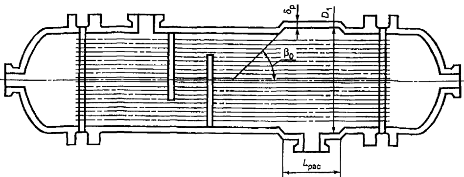
Рисунок 3 — Аппарат с расширителем на кожухе
