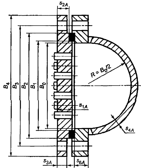
Рисунок 18 — Камера разъемной конструкции со сварной полуцилиндрической крышкой
