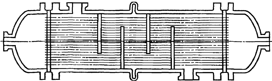
Рисунок 2 — Аппарат с компенсатором на кожухе
