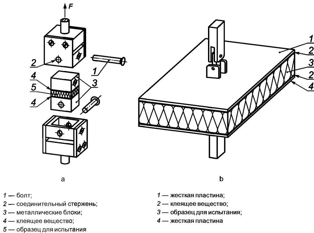
Рисунок 1 — Примеры приспособлений для крепления образца
