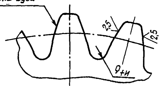
Вид Г M5:1
