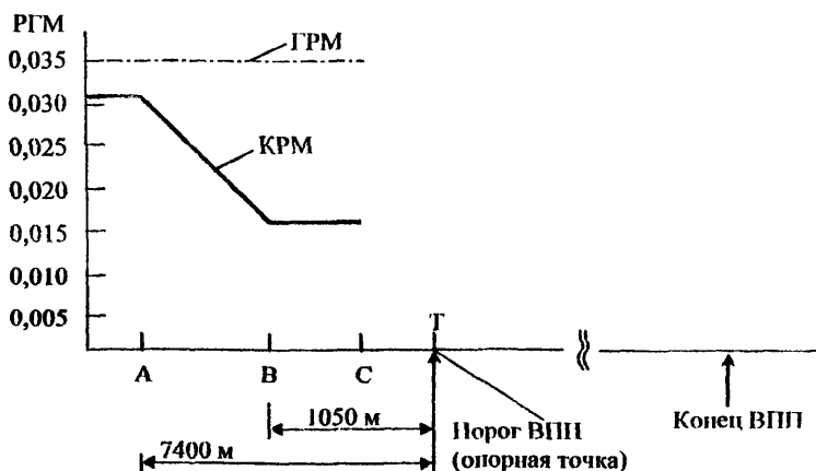
Рис. 5.5. Максимально допустимые амплитуды искривлений линий курса и глссады для КРМ и ГРМ категории I
