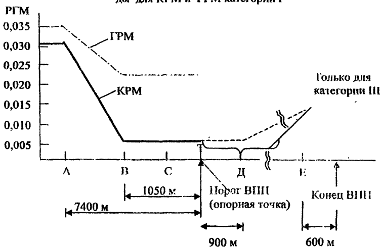
Рис. 5.5. Максимально допустимые амплитуды искривлений линий курса и глссады для КРМ и ГРМ категории I
