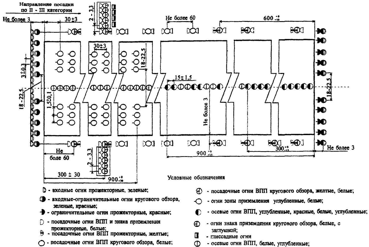
Рис. 5.16. Схема расположения огней ВПП систем точного захода на посадку II и III категории (ОВИ-II, ОВИ-III)
