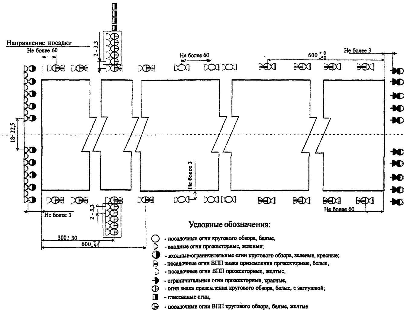
Рис. 5.13. Схема расположения огней на ВПП с одного направления посадки системы точного захода на посадку I категории (ОБИ-1)
