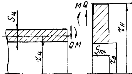
Рис.4 Узел сопряжения цилиндрической оболочки с пластиной
