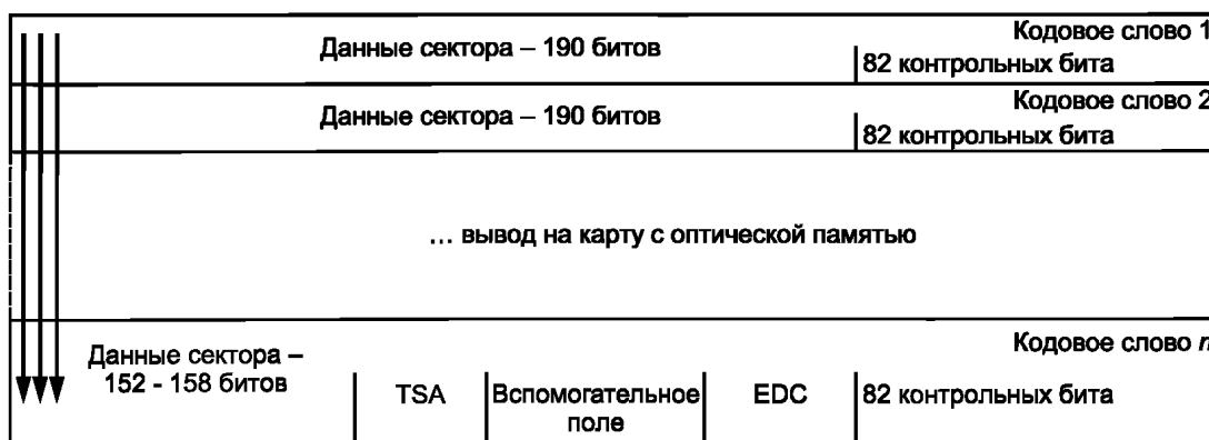
Рисунок В.13 — Перемежение данных сектора с кодом EDAC, секторы типов 0—4
