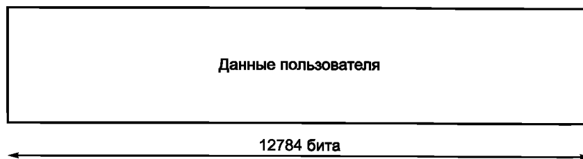
Рисунок В.11 — Структура блока данных сектора типа 5
