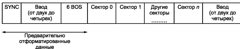
Рисунок В.5 — Структура полной дорожки, секторы типов 0—5
