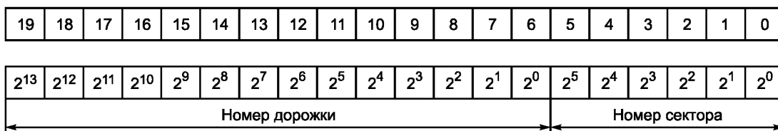
Рисунок В.4 — Формат адреса сектора и дорожки
