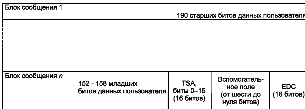
Рисунок В.12 — Данные сектора до применения кода EDAC (для секторов всех типов, за исключением типа 5)
