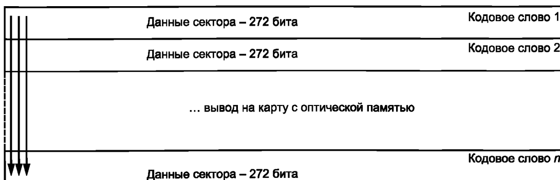
Рисунок В.14 — Перемежение данных сектора, сектор типа 5
