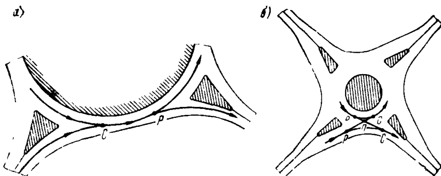
Рис 23 Схема расположения конфликтных точек на кольцевом пересечении с центральными островками
