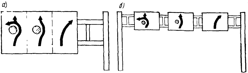
Рис 65. Разновидности знака «Направления движения по полосам» (5.81), устанавливаемого над уширенным до трех полос движением въездом на кольцевое пересечение:
