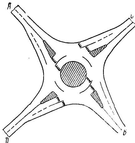
Рис. 2. Направление A—B — главное
