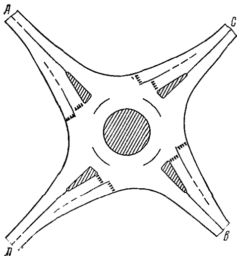
Рис. 1. Приоритет в движении на кольце
