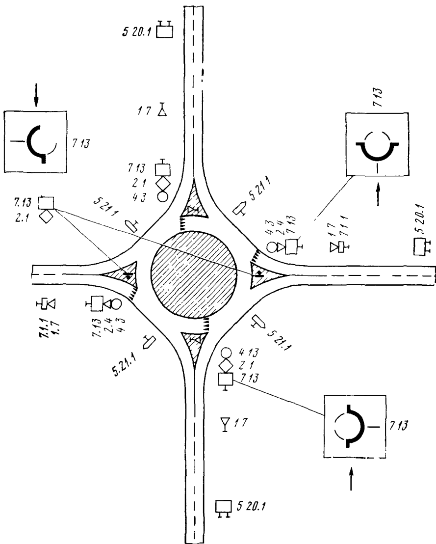
Рис. 6.2. Схема расстановки знаков на кольцевых пересечениях при прохождении главной дороги в прямом направлении
