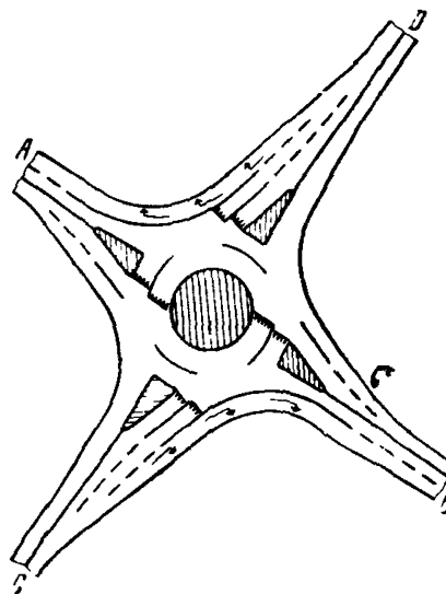
Рис 8 Направление A-B — главное; на въездах C и D имеются СПП
