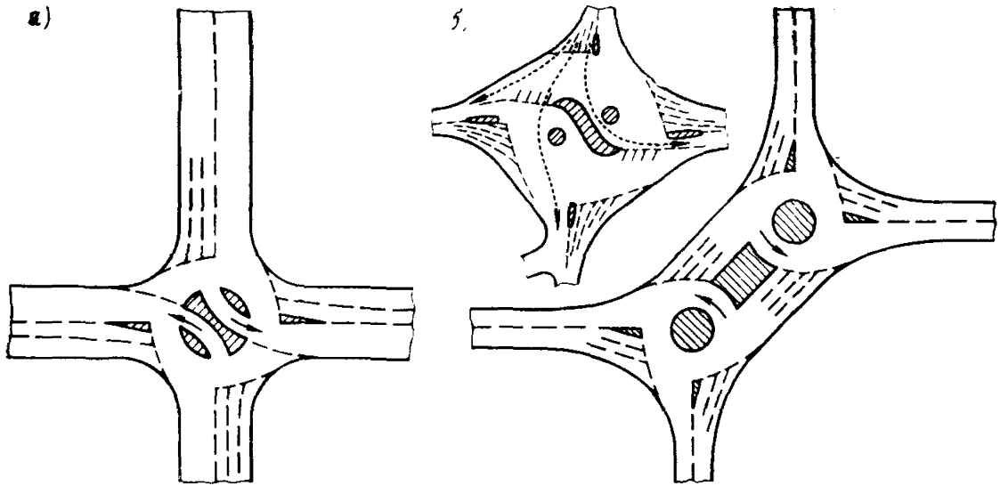
Рис 15 Планировка кольцевых пересечений со сложными центральными островками
