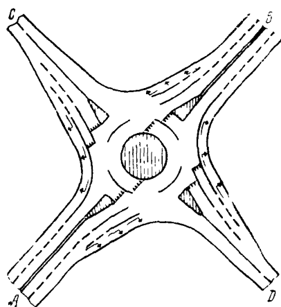
Рис 12 Направление А—В—главное, на въездах С и D имеются СПП
