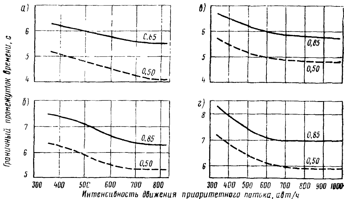
Рис 37 Изменение величины критического промежутка времени от интенсивности движения приоритетного потока
