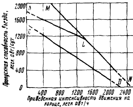
Рис. 5.1 Зависимость пропускной способности въезда на кольцевое пересечение от интенсивности движения на кольце.
