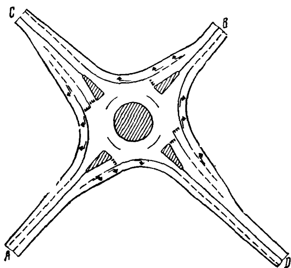
Рис. 7. Приоритет в движении на кольце; на всех въездах имеются СПП
