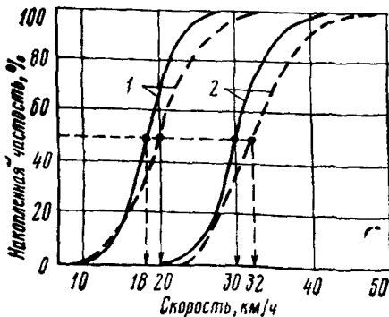
Рис 3.3 Кумулятивные кривые скоростей движения автомобилей на кольцевой проезжей части
