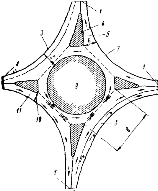
Рис 11. Элементы кольцевого пересечения
