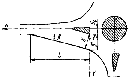
Рис. 4 3. Схема уширения участка въезда на кольцевое пересечение
