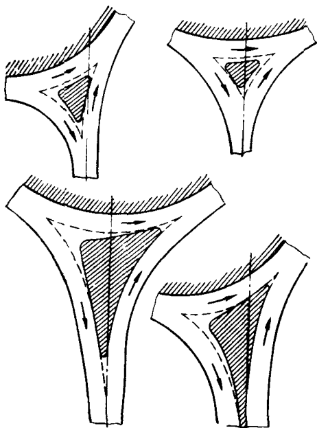
Рис 4.2 Виды направляющих островков кольцевых пересечений автомобильных дорог
