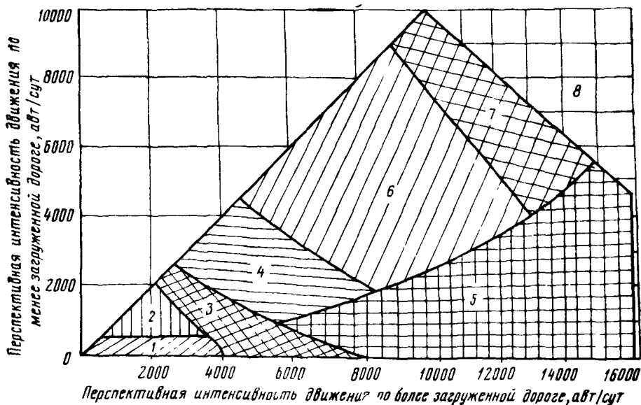
Рис 1.7 Номограмма для выбора типа планировочных решений пересечений
