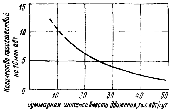
Рис 21 Распределение дорожно-транспортных происшествий на кольцевом пересечении
