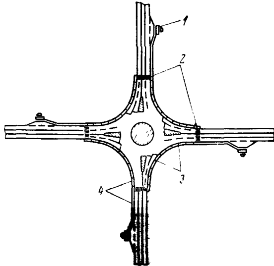
Рис 24 Схема организации пешеходного движения на кольцевом пересечении
