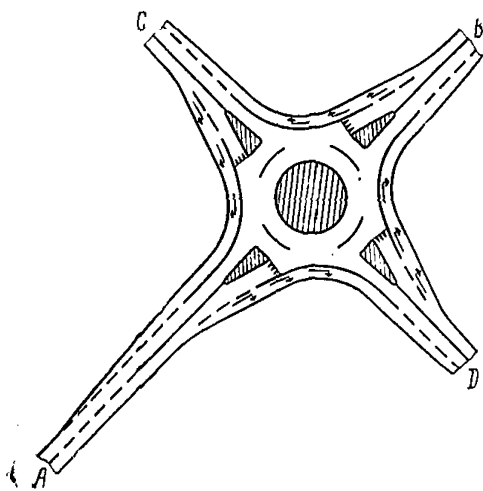
Рис. 3. Приоритет в движении на кольце; на всех въездах имеются специальные правоповоротные полосы (СПП)
