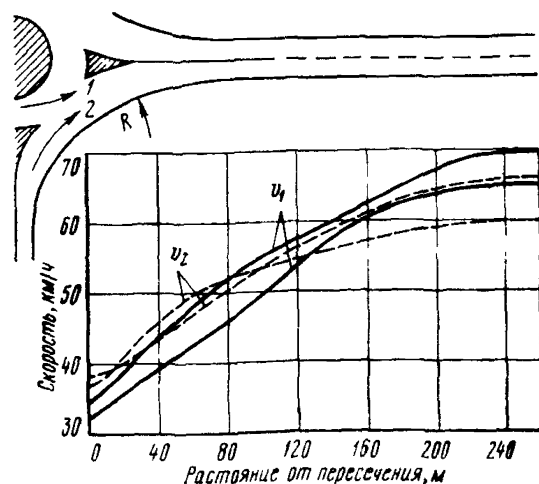
Рис 45 Характер изменения скорости движения на участке выезда из кольцевого пересечения при D_{до}=42 м, R=25 м
