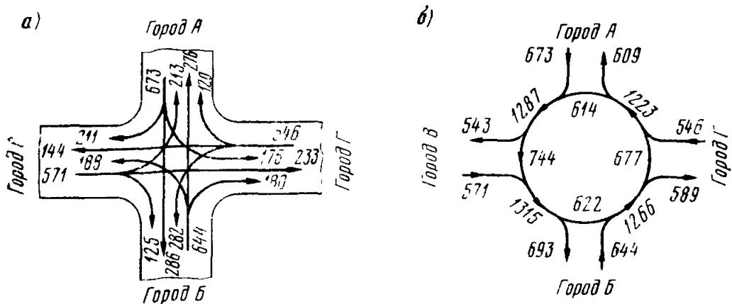
Рис 31 Картограмма интенсивности (авт/ч) движения на кольцевом пересечении:
