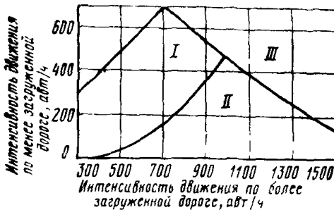
Рис 66. Номограмма для выбора варианта организации движения на кольцевых пересечениях.
