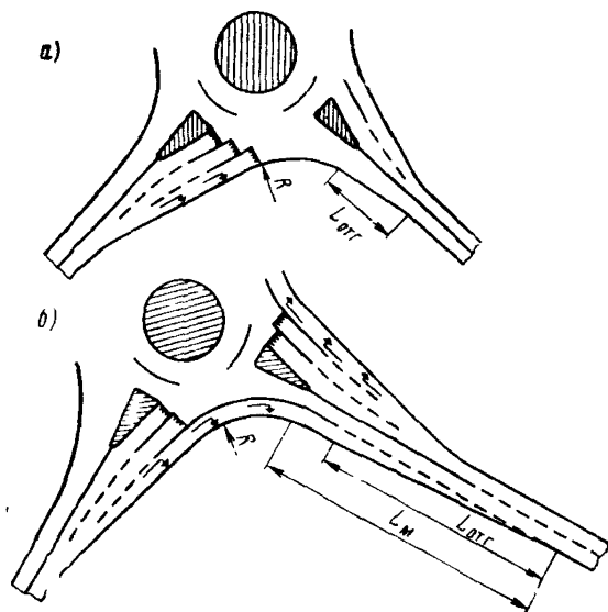
Рис 44 Схема уширения на участке выезда кольцевого пересечения:
