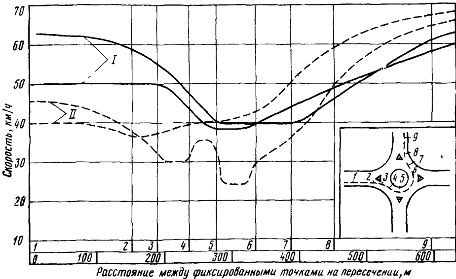
Рис. 35. Изменение скорости движения на кольцевом пересечении неравнозначных дорог с виражом на кольцевой проезжей части при левопоротном проезде:
