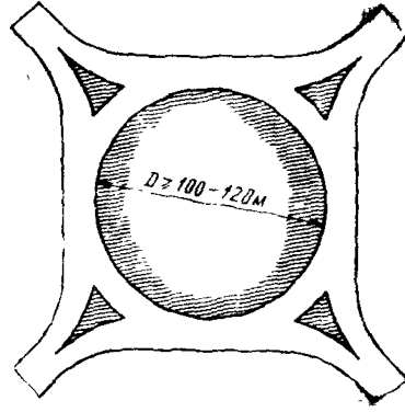
Рис 13 Кольцевое пересечение с центральным островком малого диаметра.
