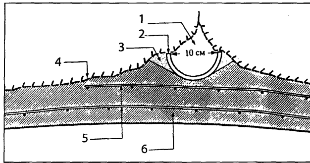
Рис.8.1. Пример устройства водоотвода (дрены) за пределы покрытия из торкрет-бетона. 1 – дрена; 2 – желоб; 3 – быстросхватывающийся раствор; 4 – скальная порода; 5 – арматурная сетка; 6 – торкрет-бетон.
