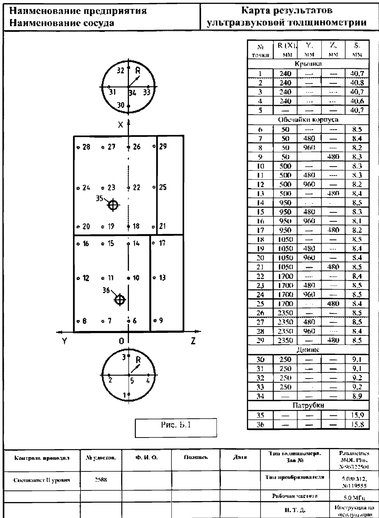
Рис. Б.1. Пример карты результатов ультразвуковой толщинометрии
