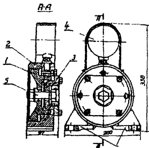
Рисунок 1В - Общий вид устройства УТБ-40
